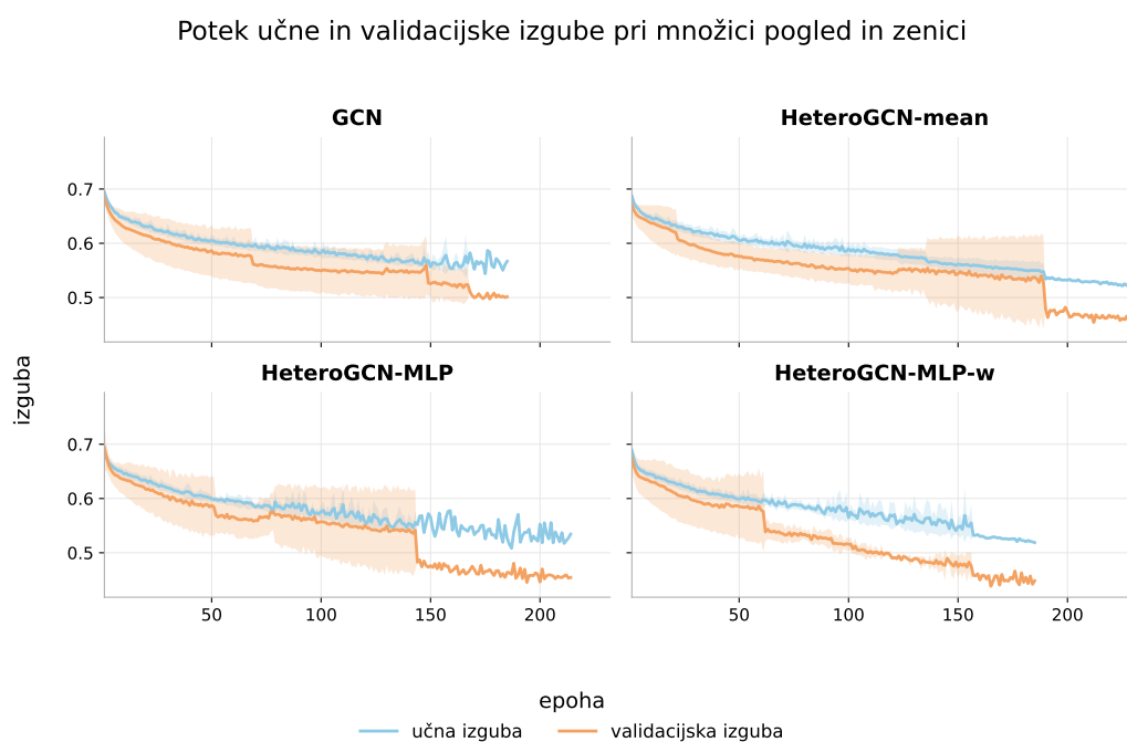
Slika 6.1: Povprečni potek učne in validacijske izgube grafovskih modelov pri množici signalov pogled in zenici . Zasenčena območja predstavljajo standardni odklon čez sedem delitev po subjektih.
