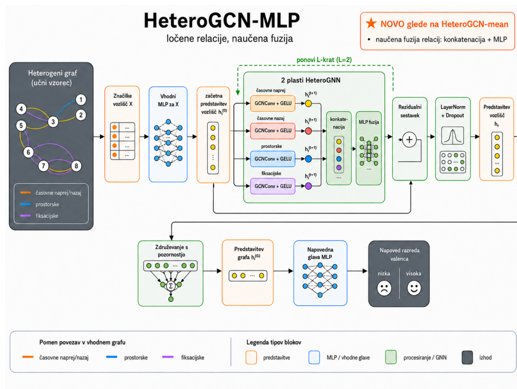
Slika 6.3: Diagram arhitekture HeteroGCN-MLP. Model relacijske predstavitve najprej konkatenera, nato pa jih združi z naučeno fuzijo prek dvoslojnega perceptrona.
