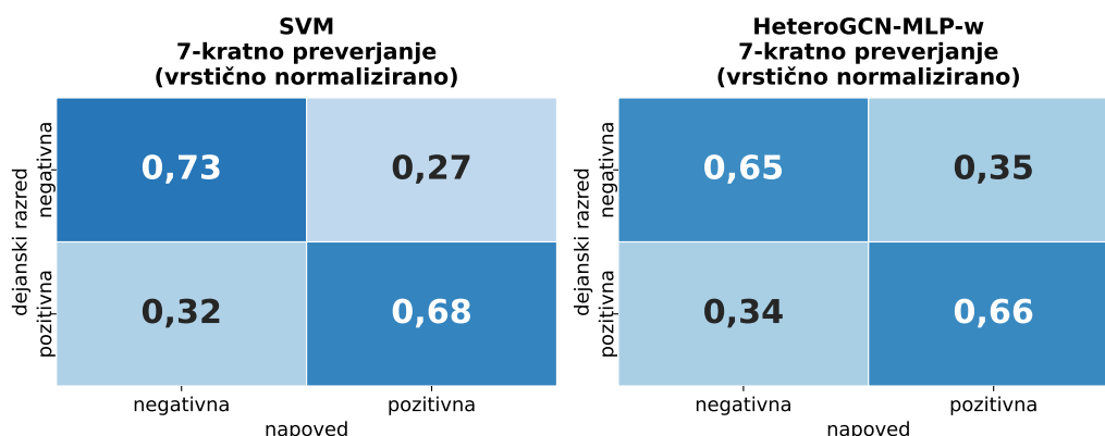
Slika 7.2: Vrstično normalizirani matriki zamenjav za najboljši model SVM in najboljši grafovski model HeteroGCN-MLP-w pri množici signalov pogled in zenici .
