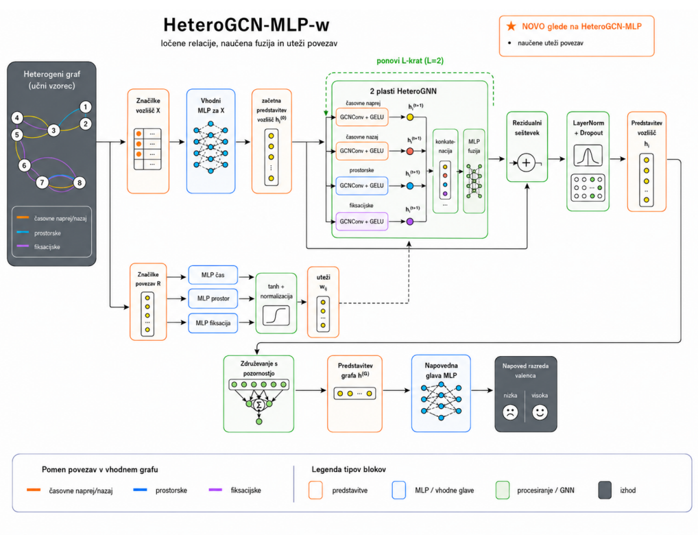
Slika 5.4: Diagram arhitekture HeteroGCN-MLP-w. Model poleg učljive fuzije relacij uporablja še značilke povezav, iz katerih z relacijsko odvisnimi perceptroni izračuna učljive predznačene uteži povezav.
