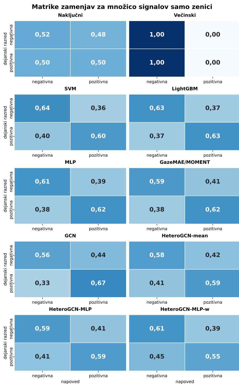
Slika A.2: Matrike zamenjav za množico signalov samo zenici . Razporeditev modelov je enaka kot pri drugih množicah signalov: izhodiščna modela, trije klasični oziroma nevronske primerjalni modeli, zamrznjene predstavitve in štiri grafovske arhitekture.
