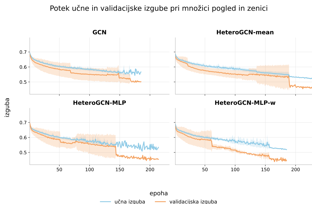
Slika 7.1: Povprečni potek učne in validacijske izgube grafovskih modelov pri množici signalov pogled in zenici . Zasenčena območja predstavljajo standardni odklon čez sedem delitev po subjektih.
