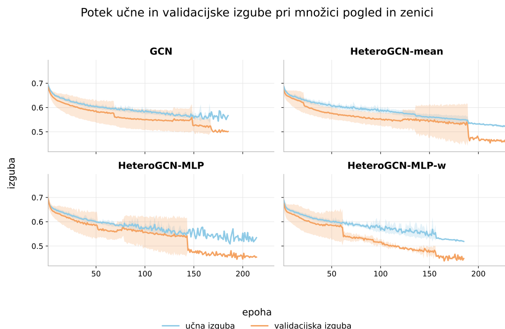
Slika 8.1: Povprečni potek učne in validacijske izgube grafovskih modelov pri množici signalov pogled in zenici . Zasenčena območja predstavljajo standardni odklon čez sedem delitev po subjektih.
