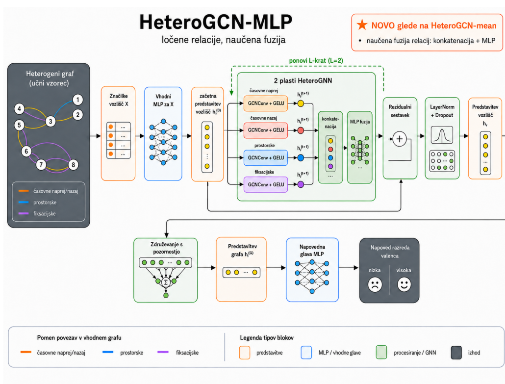
Slika 6.3: Diagram arhitekture HeteroGCN-MLP. Model relacijske predstavitve najprej konkatenira, nato pa jih združi z naučeno fuzijo prek dvoslojnega perceptrona.
