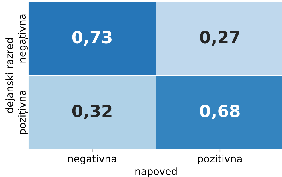
SVM 7-kratno preverjanje (vrstično normalizirano)
