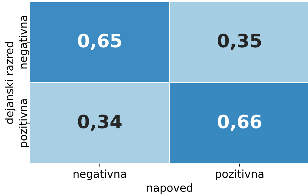
HeteroGCN-MLP-w 7-kratno preverjanje (vrstično normalizirano)
