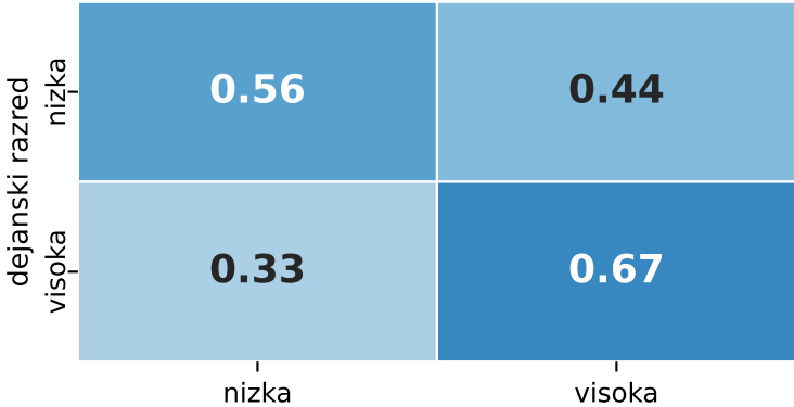
HeteroGCN-MLP
