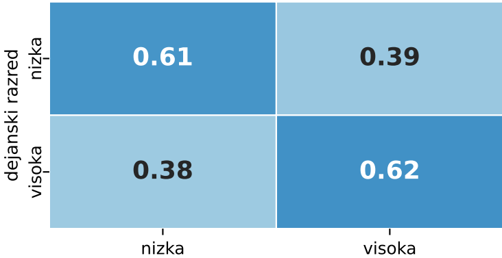
GCN
