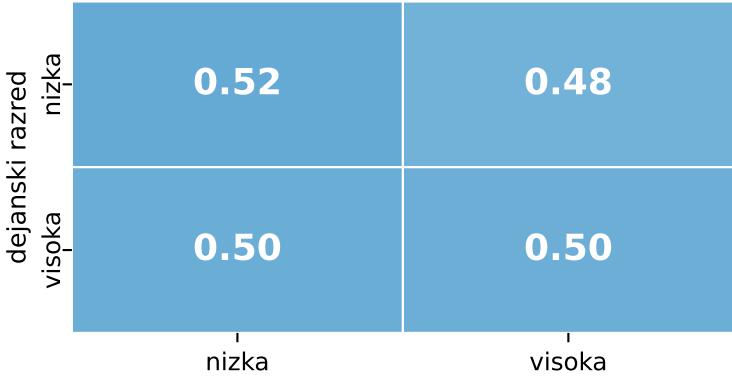
SVM
