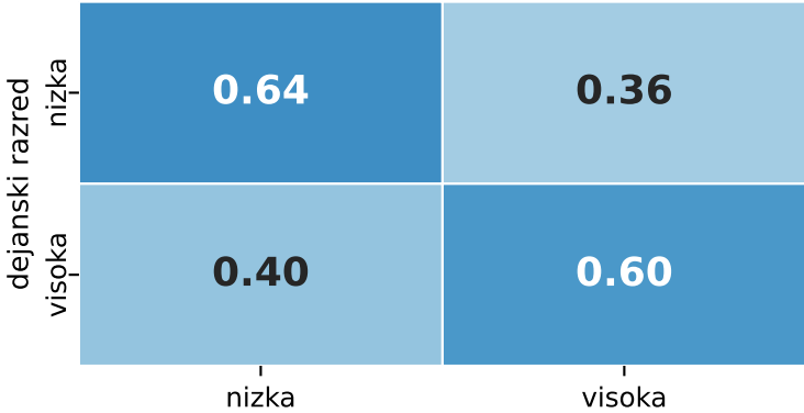
MLP
