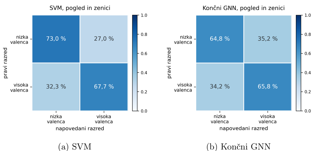
Slika 8.3: Vrstično normalizirani matriki zmede za najboljši model in najboljši grafovski model pri množici signalov pogled in zenici.
