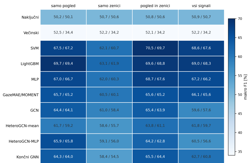
Slika 8.2: Toplotni prikaz glavne primerjave modelov. V celicah sta zapisani točnost / makro F1 v odstotkih, barva pa prikazuje makro F1.
