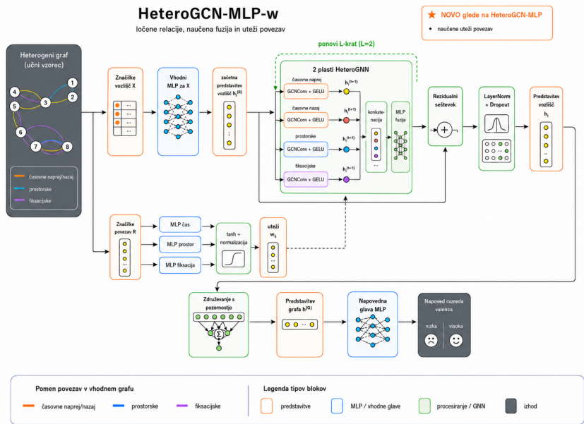
Slika 6.4: Diagram arhitekture HeteroGCN-MLP-w . Model poleg naučene fuzije relacij uporablja še značilke povezav, iz katerih z relacijsko odvisnimi perceptroni izračuna naučene predznačene uteži povezav.
