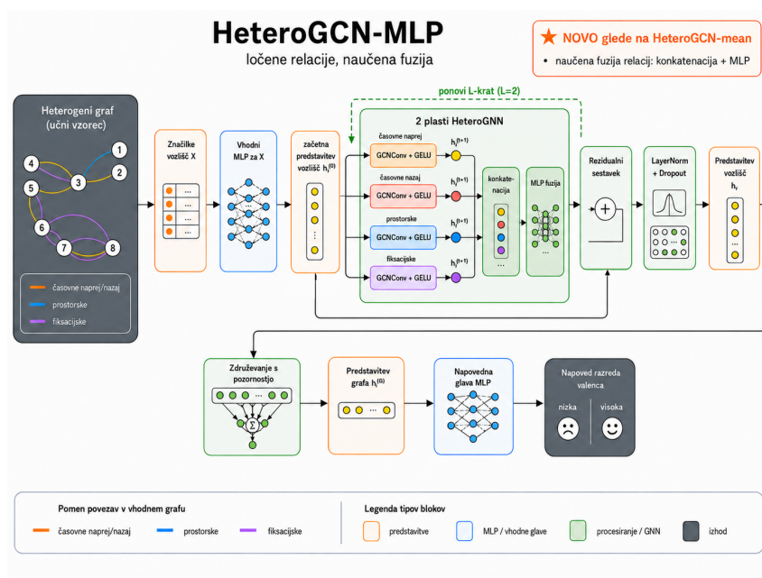
Slika 6.3: Diagram arhitekture HeteroGCN-MLP . Model relacijske predstavitve najprej konkatenerira, nato pa jih združi z naučeno fuzijo prek dvoslojnega perceptrona.
