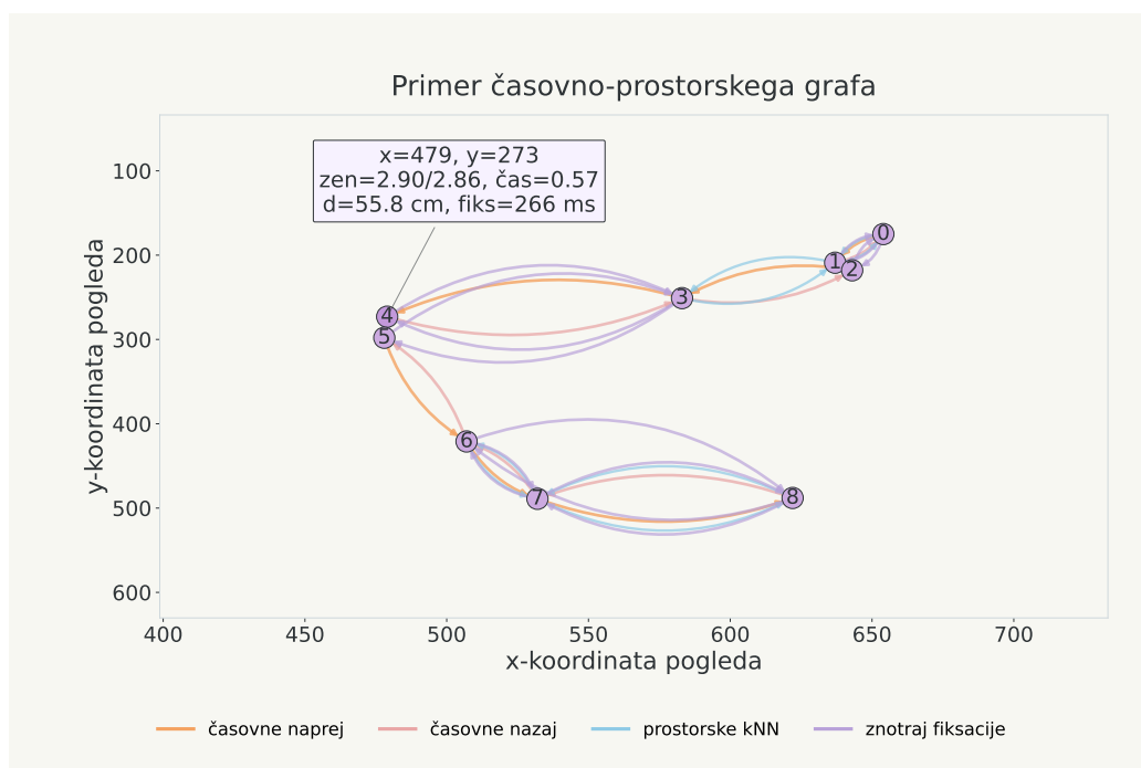
Slika 5.2: Primer grafovske konstrukcije za množico usi signali . Vozlišča predstavljajo meritve v izseku časovnega okna, povezave pa prikazujejo časovne, prostorske in fiksacijske relacije. Ločeni prikazi posameznih relacij so zbrani v dodatku C.
