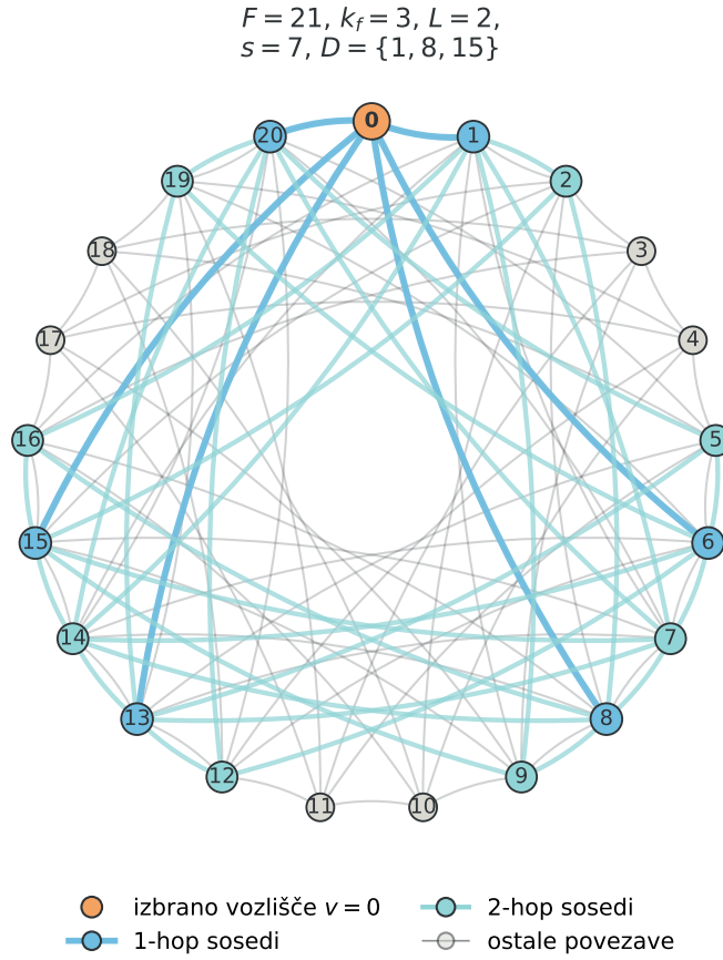
Slika 5.1: Shematski prikaz razširjenih povezav znotraj ene fiksacije za povprečno velikost fiksacije. Iz F = 21 in k_f = 3 izračunamo s = 7 in D = \{1, 8, 15\} . Število plasti GNN je L = 2 , kar vpliva na doseg sporočila posameznega vozlišča in gostoto grafa. Vozlišča so prikazana v krogu z lokalnimi indeksi znotraj fiksacije. Odtenka modrih povezav ločita neposredne sosede izbranega vozlišča v = 0 in dodatna vozlišča, dosegljiva v drugem skoku po fiksacijski relaciji.
