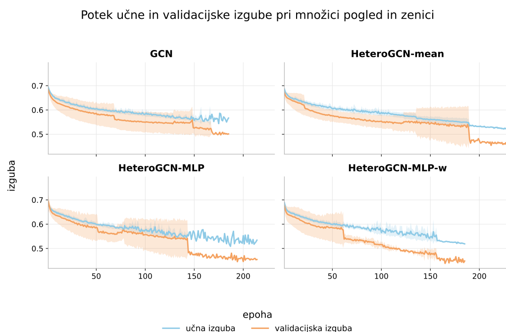
Slika 8.1: Povprečni potek učne in validacijske izgube grafovskih modelov pri množici signalov pogled in zenici . Zasenčena območja predstavljajo standardni odklon čez sedem delitev po subjektih.
