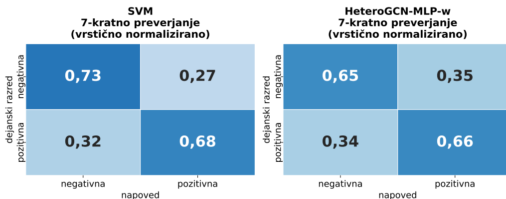
Slika 6.2: Vrstično normalizirani matriki zamenjav za najboljši model SVM in najboljši grafovski model HeteroGCN-MLP-w pri množici signalov pogled in zenici .
