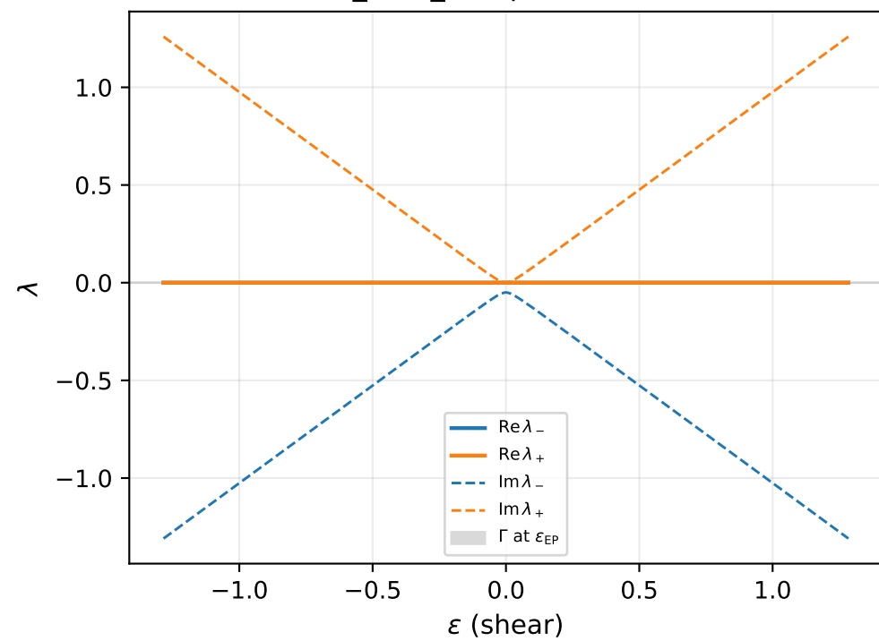
Puisseux
