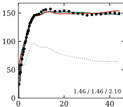
IC2574
