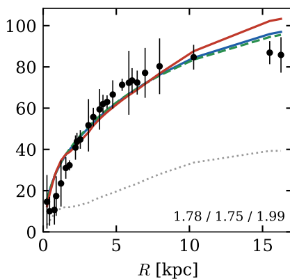
F583-1
