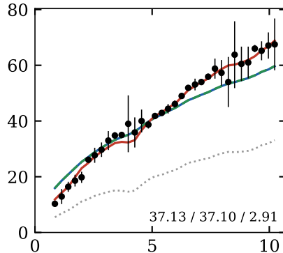
F583-1
