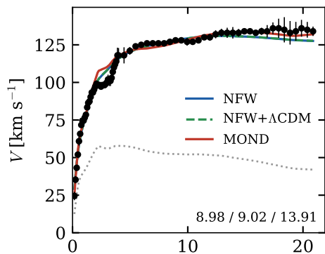
DDO154
