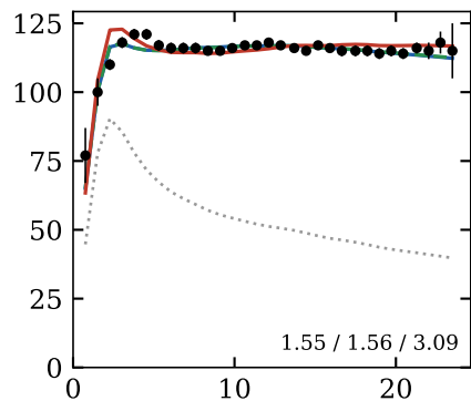
UGC00128
