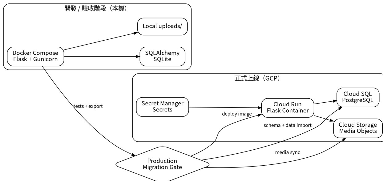
圖 2. v1.2 Local-first 到 Cloud Run 的目標架構：應用層保持不變，資料庫與媒體儲存依環境切換。
