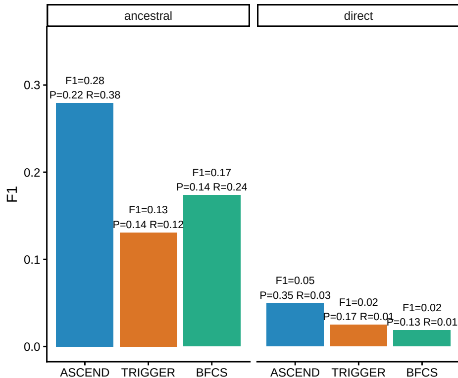
Edge-level F1 by estimand
