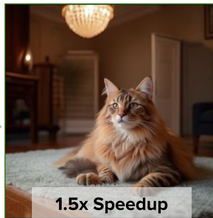
FLUX.2 Klien
