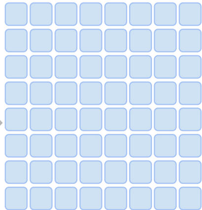
Sparse Context
