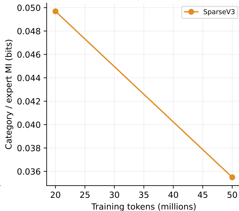
Layer 5
