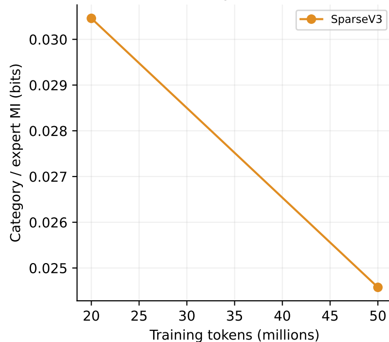
Layer 2
