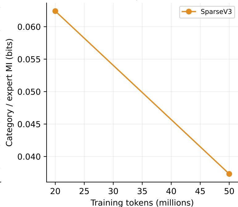
Layer 8
