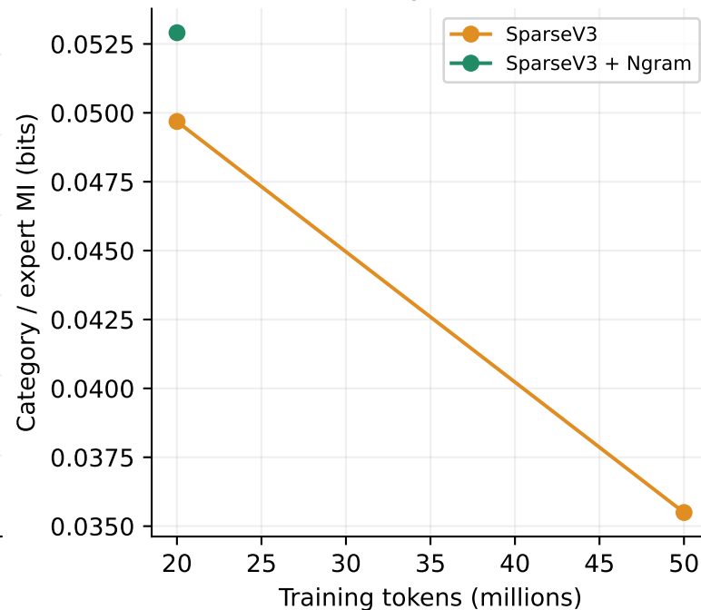
Layer 5
