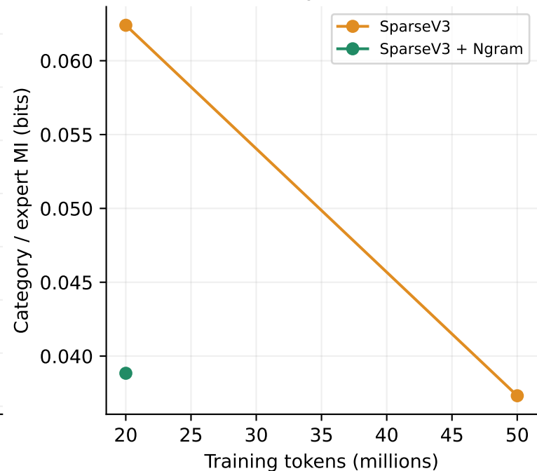
Layer 8
