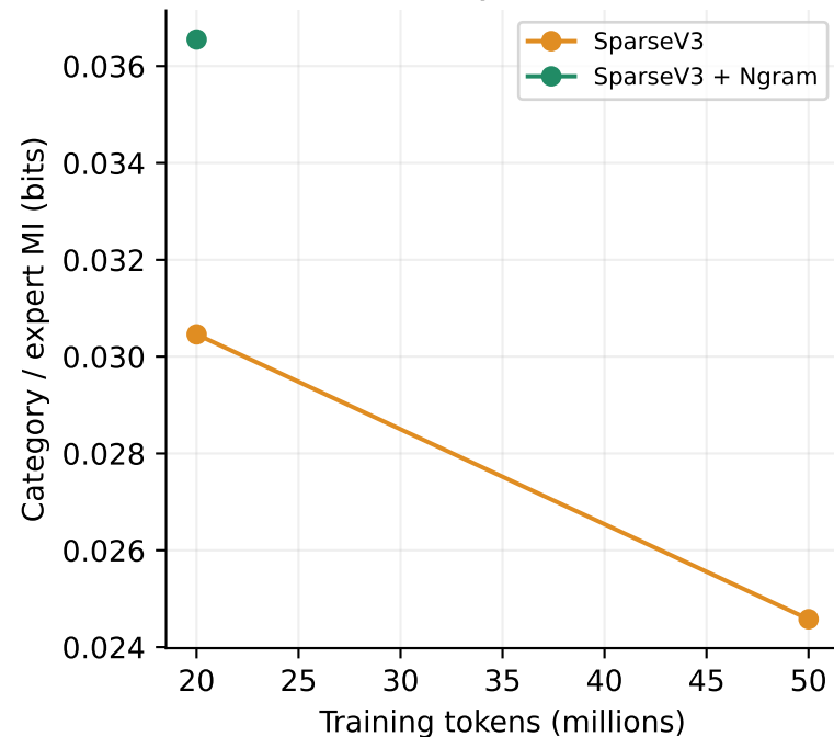
Layer 2
