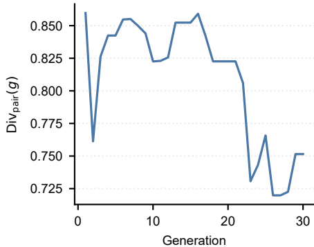
Population diversity
