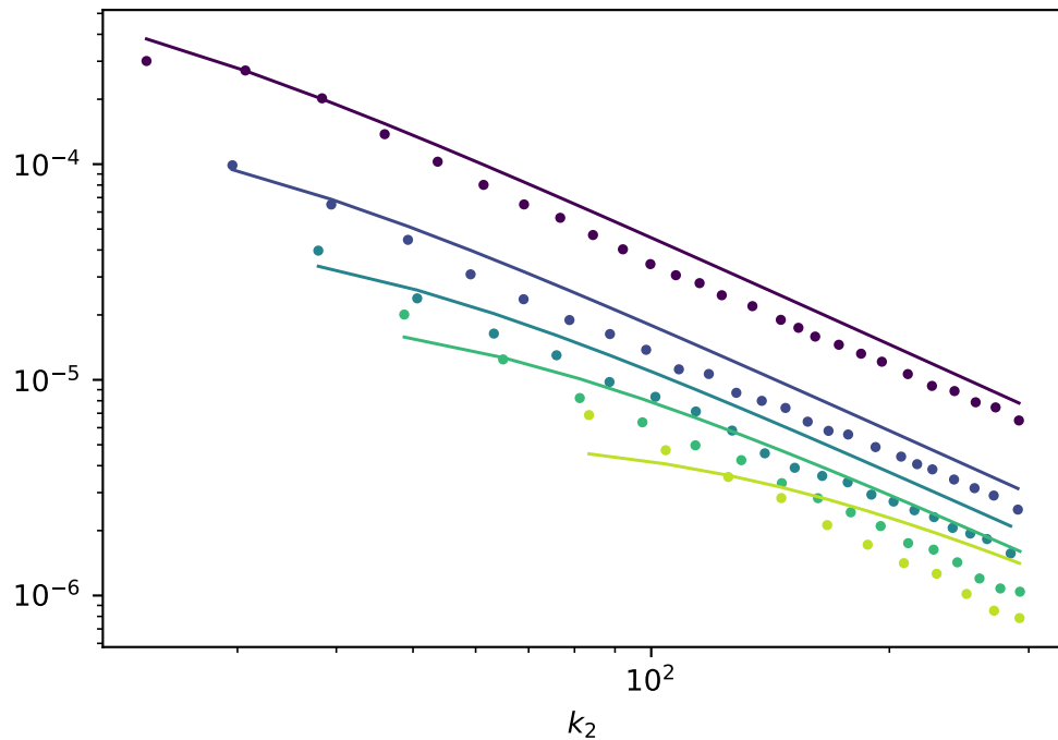
E_{\perp} : data + RDT-vK fit
