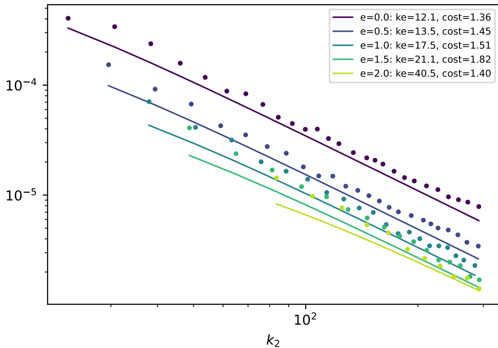
E_2 : data + RDT-vK fit
