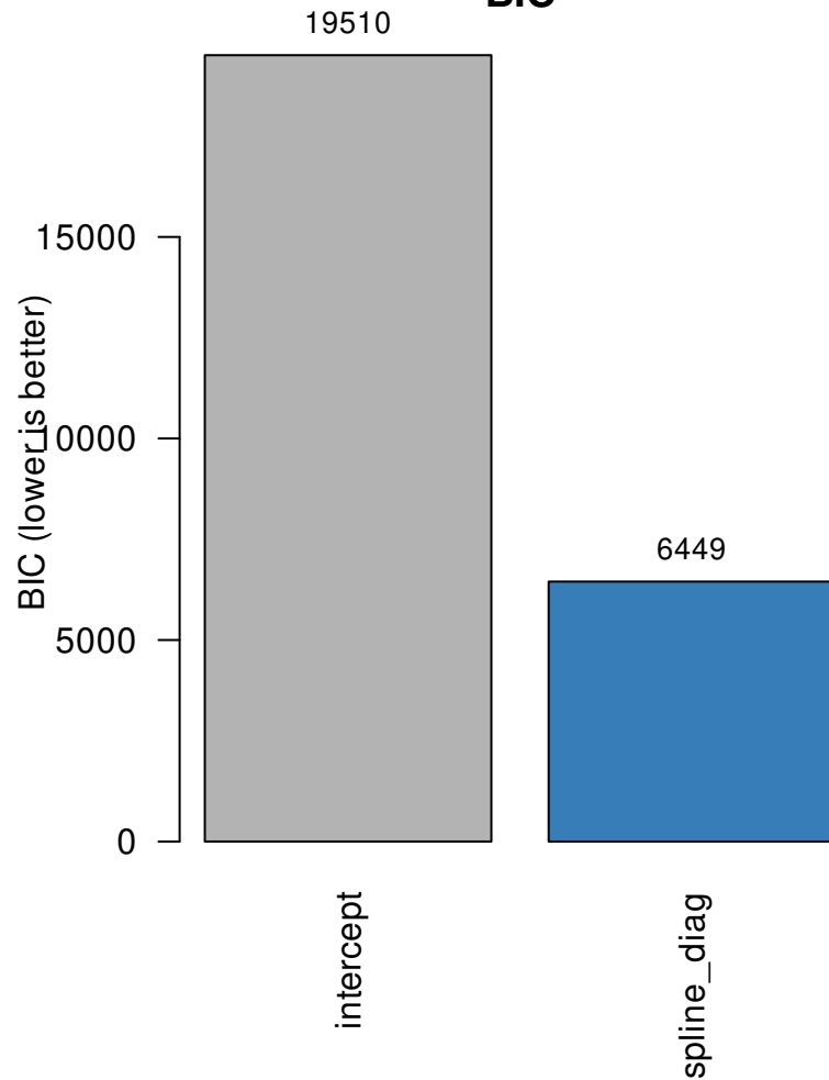
BIC
