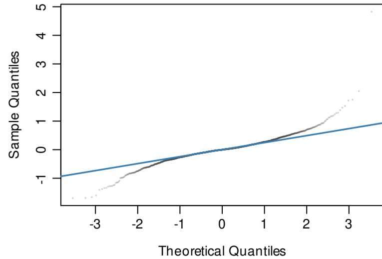
normal Q-Q
