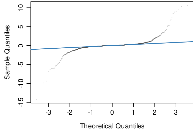
normal Q-Q
