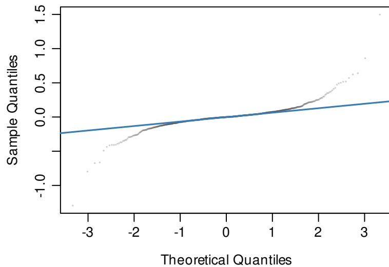
normal Q-Q
