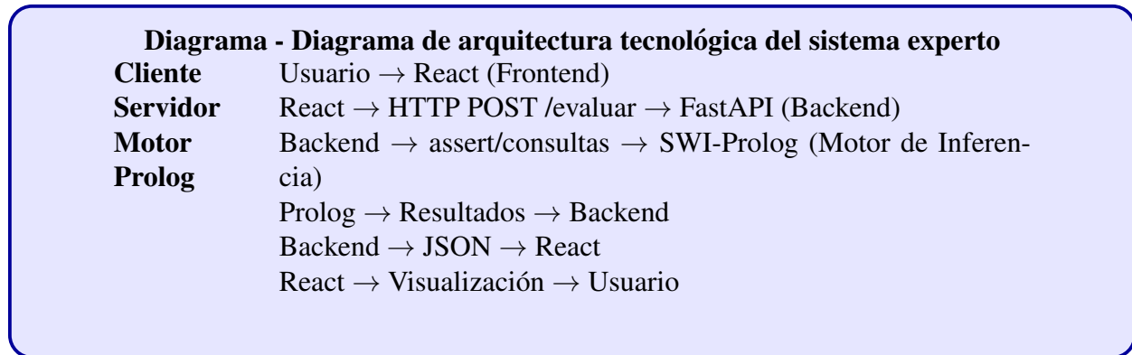
Figura 9: Diagrama de arquitectura tecnológica del sistema experto
