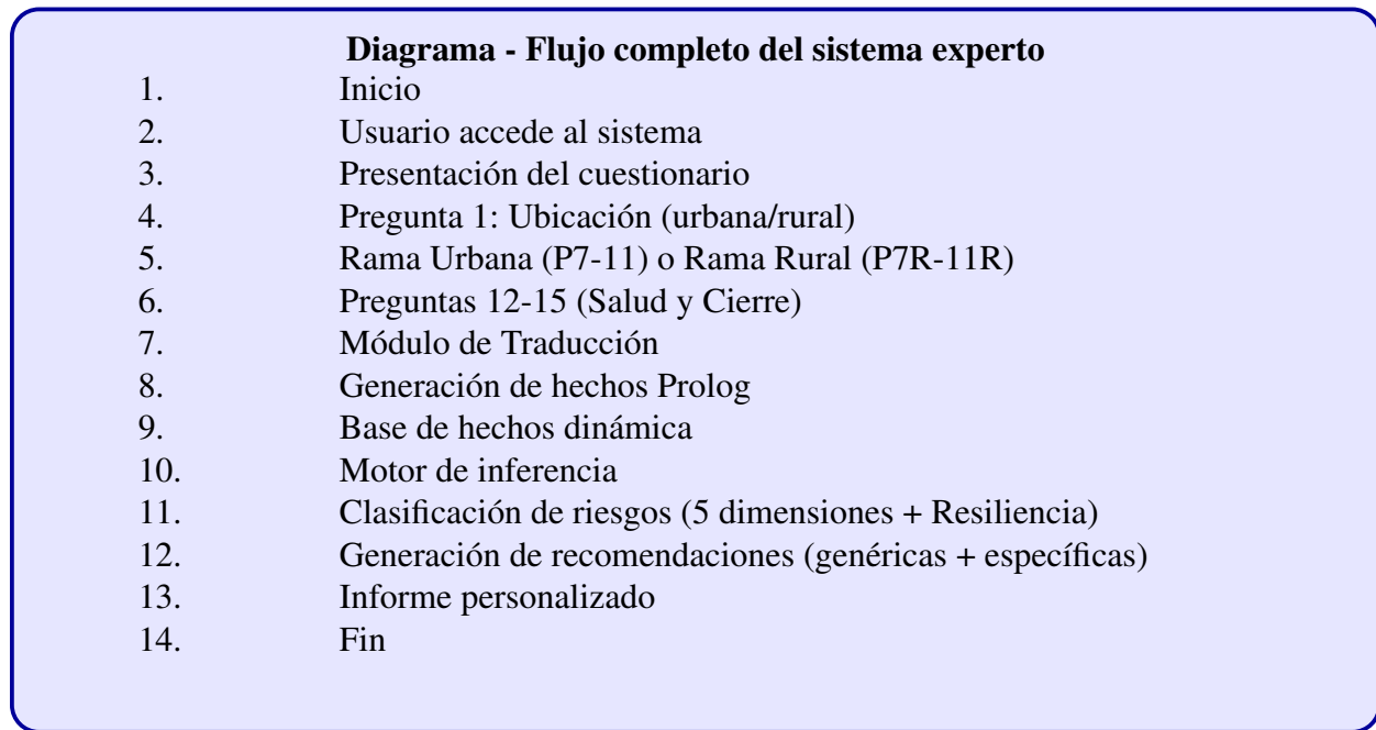
Figura 7: Flujo completo del sistema experto
