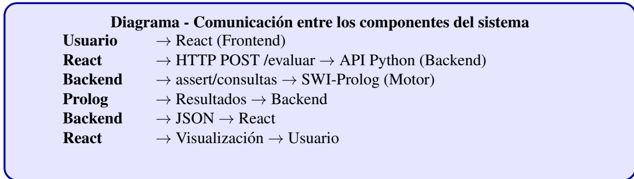
Figura 8: Comunicación entre los componentes del sistema
