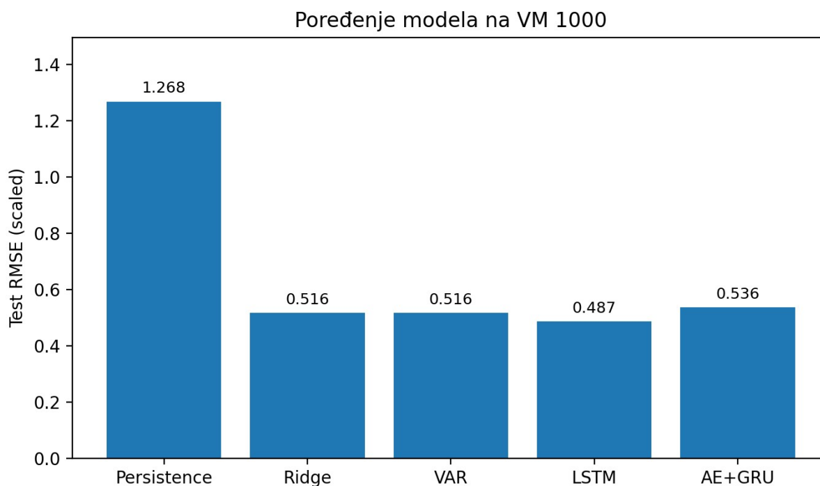
Slika 1. Test RMSE u standardizovanom prostoru za sve razmatrane modele.
