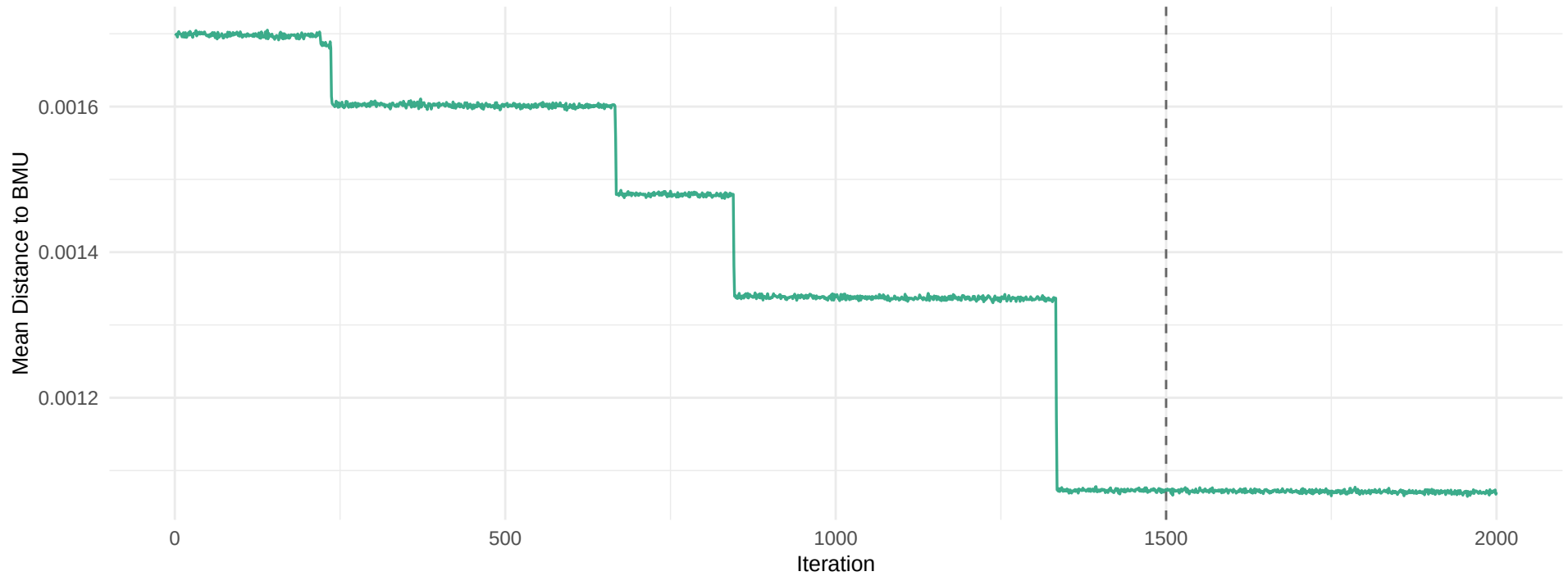
SOM Training Convergence (Selected Model)
