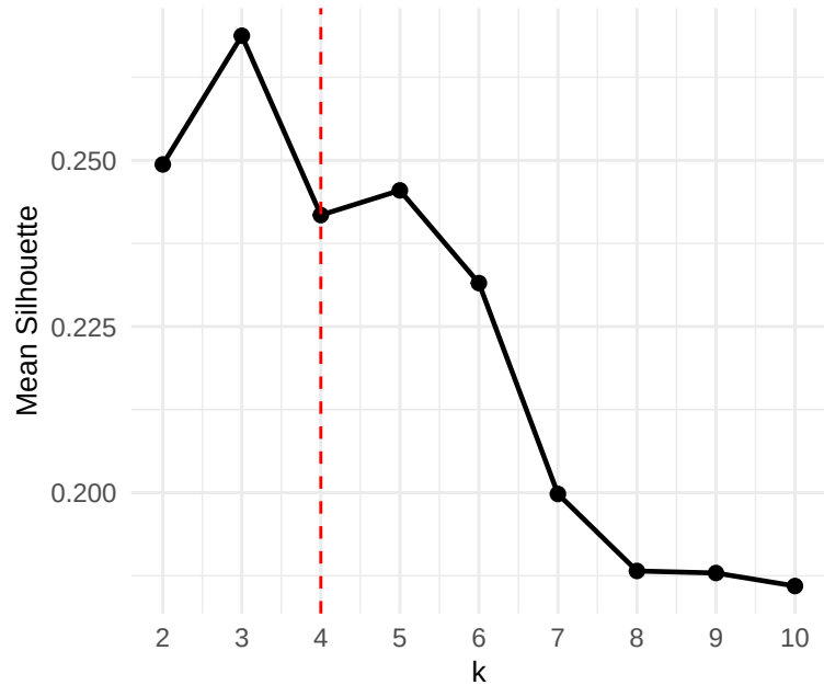
Silhouette Width
