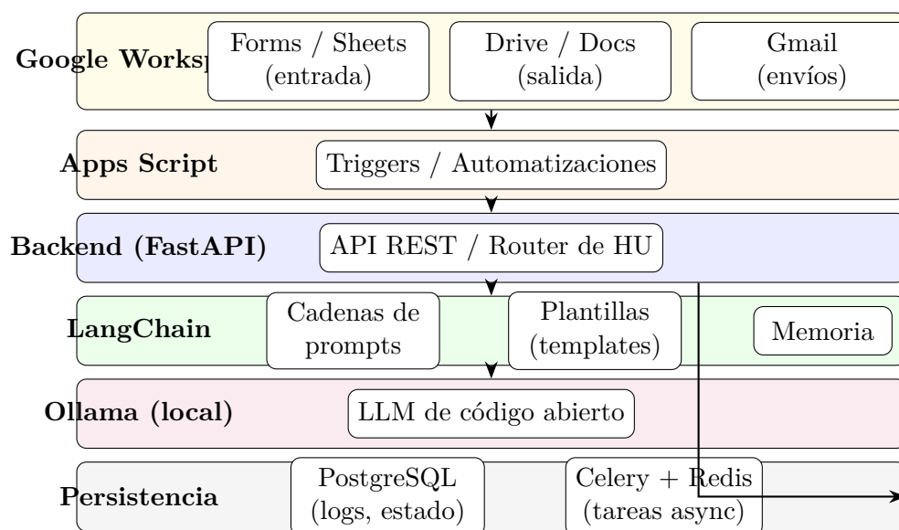
Figura 3: Arquitectura de componentes del Agente 1 (Extensión Bot)
