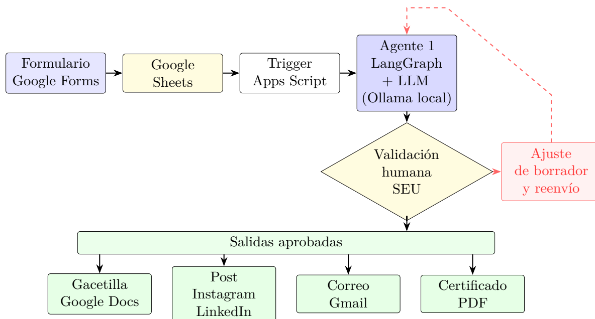
Figura 2: Flujo principal del Agente 1 (Extensión Bot): desde el ingreso de datos hasta la publicación final, con validación humana obligatoria. La publicación es manual y la realiza el personal de la SEU; la única entrega automática del agente es el correo de confirmación de inscripción (HU-012), posterior a la aprobación.
