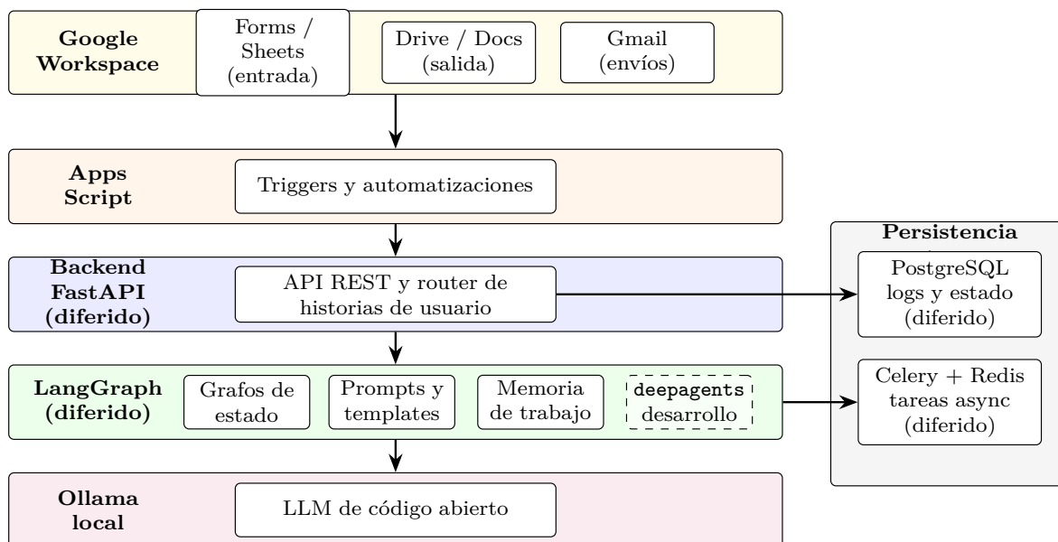
Figura 3: Arquitectura de componentes del Agente 1 (Extensión Bot). Los componentes marcados como diferidos (FastAPI, LangGraph, Celery, Redis, PostgreSQL) corresponden a la arquitectura objetivo y no están en uso al corte de este documento; ver nota en §13
