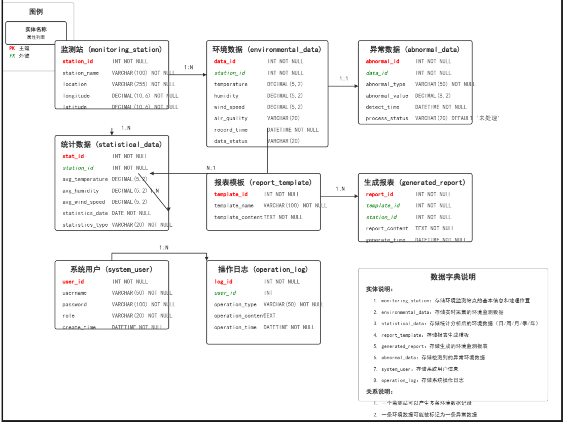
环境监测系统数据库实体关系图
