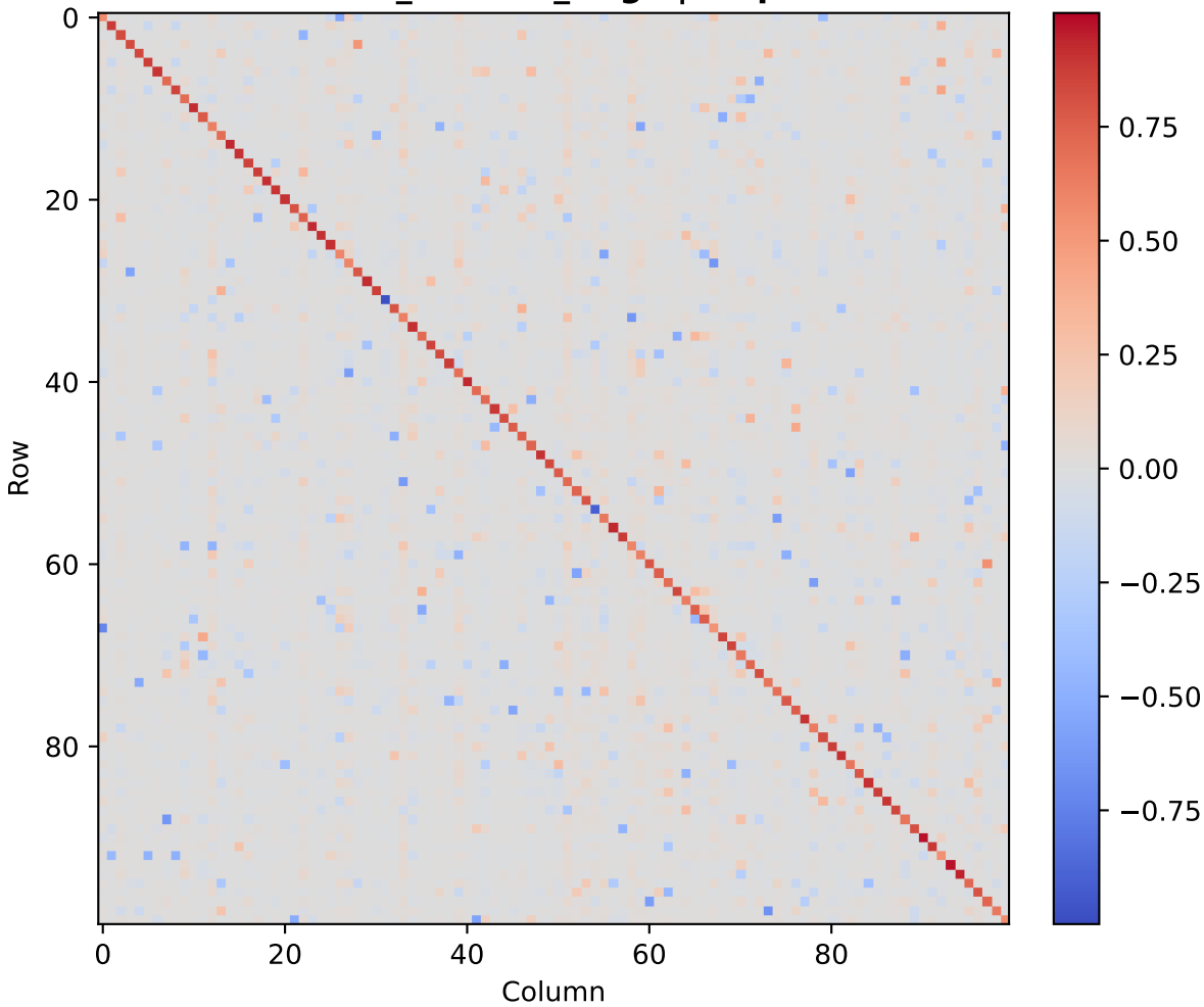
muon_random_large | step 3
