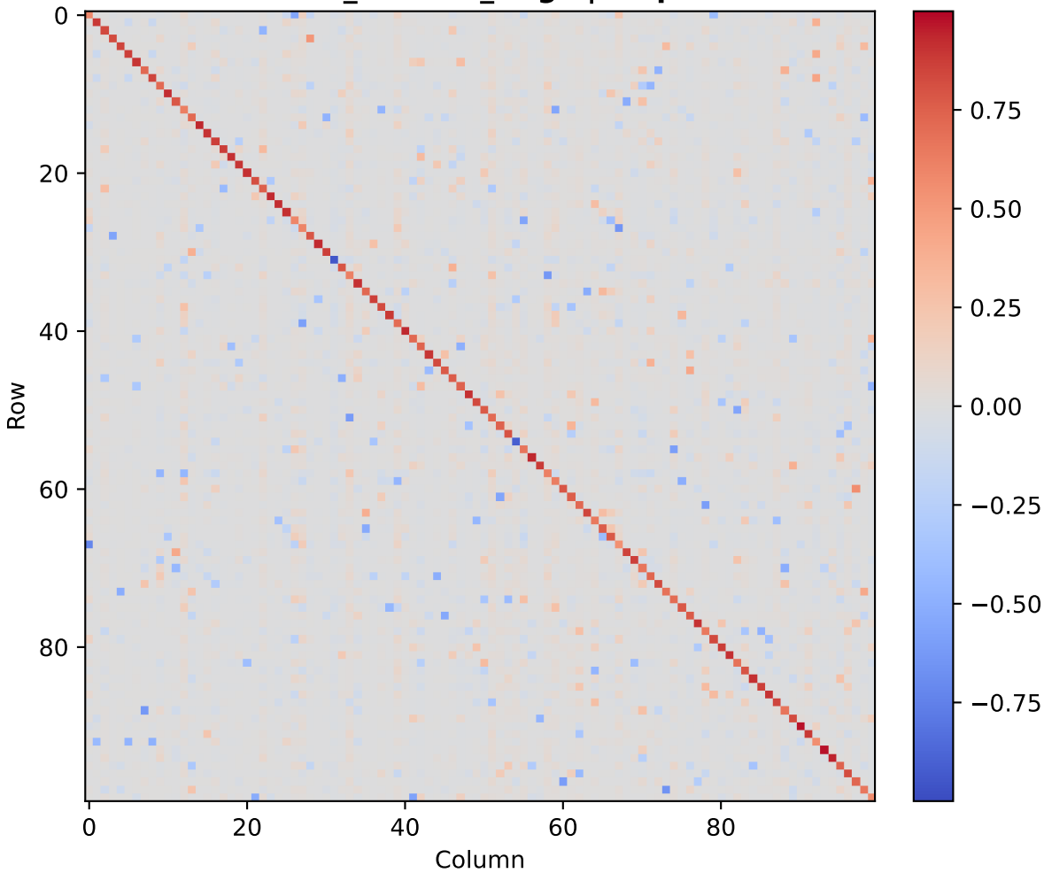
muon_random_large | step 4
