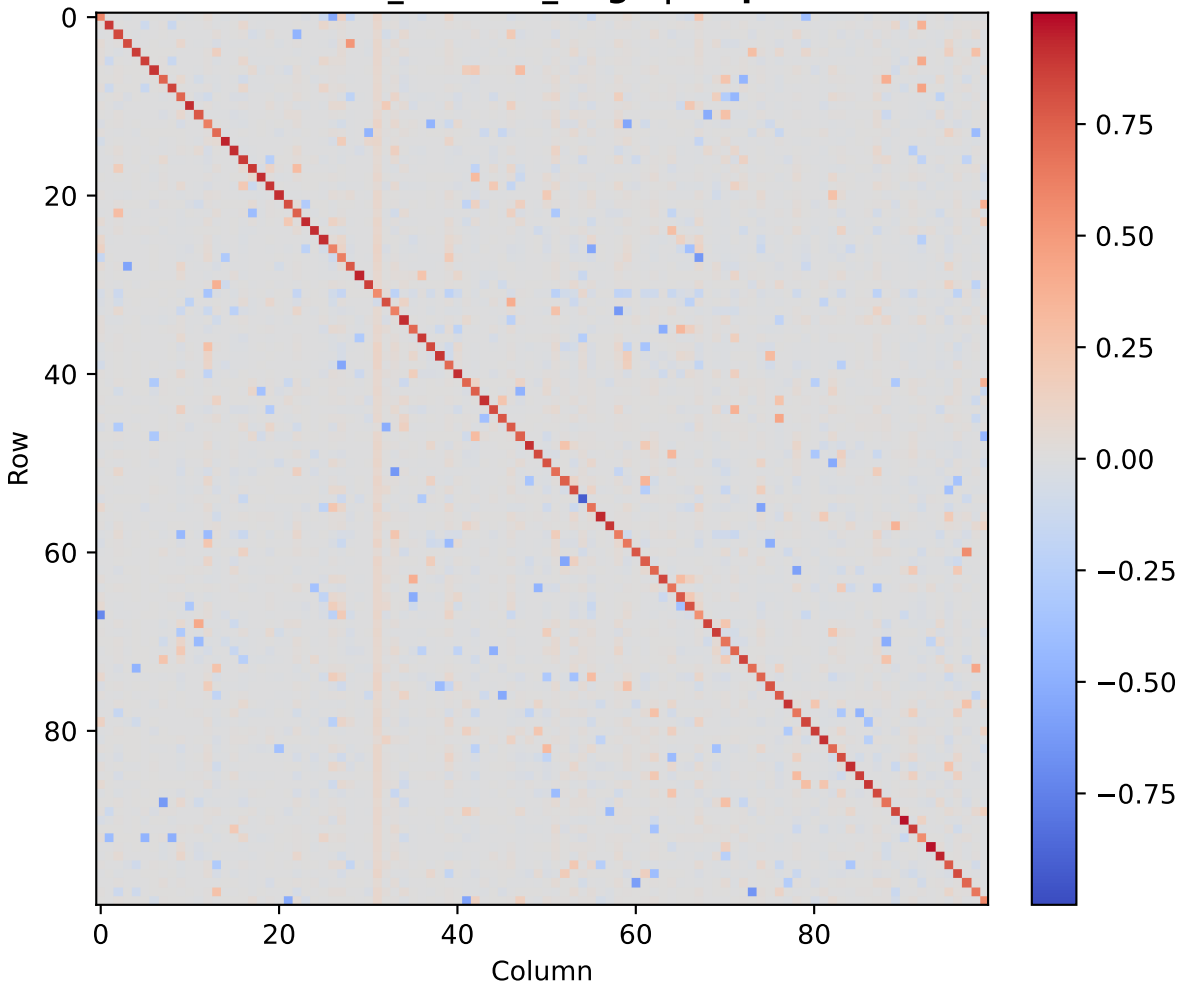
muon_random_large | step 6
