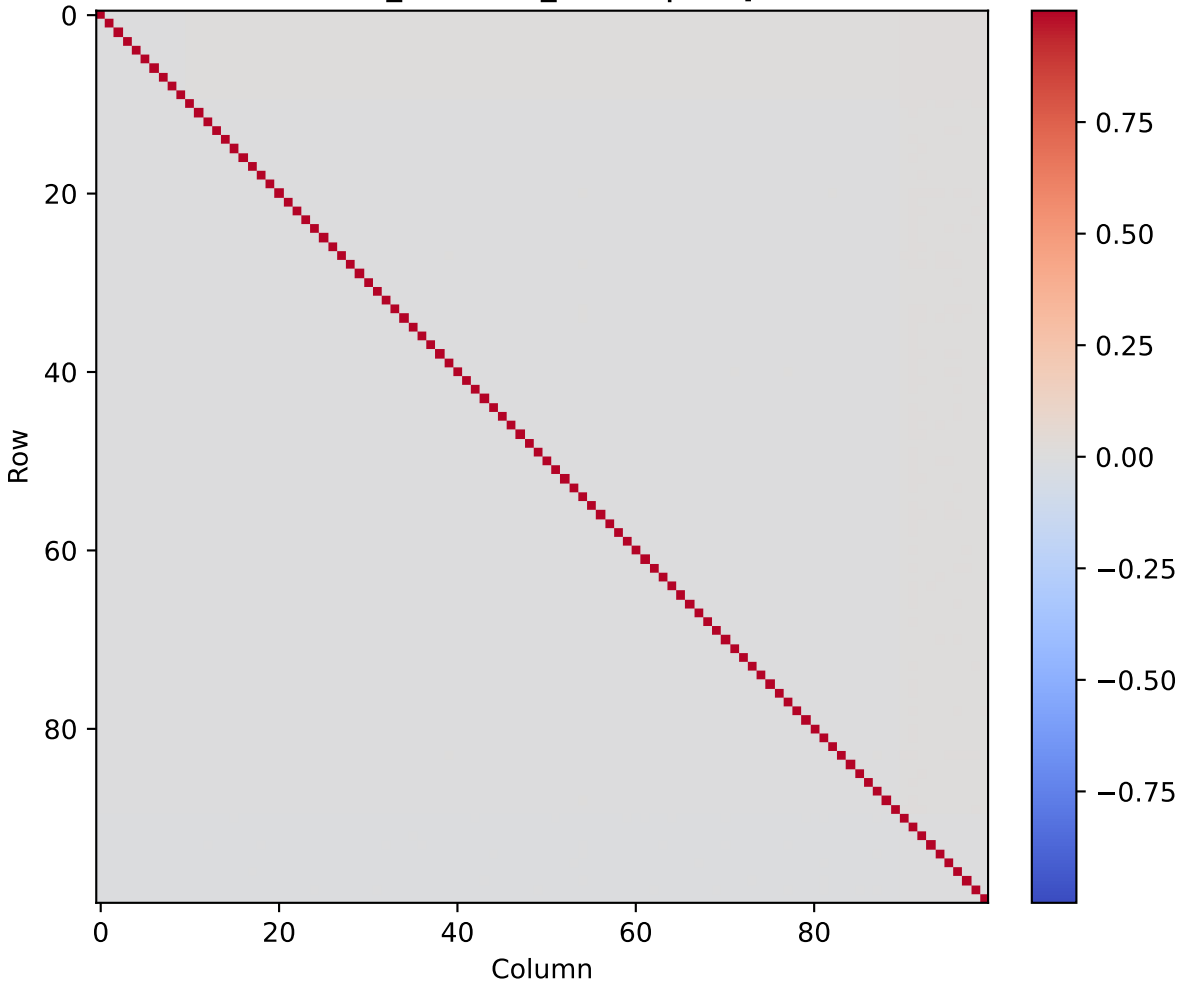
muon_random_small | step 9
