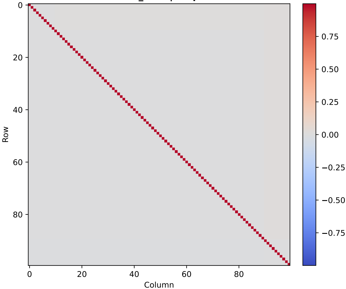
muon_zero | step 3
