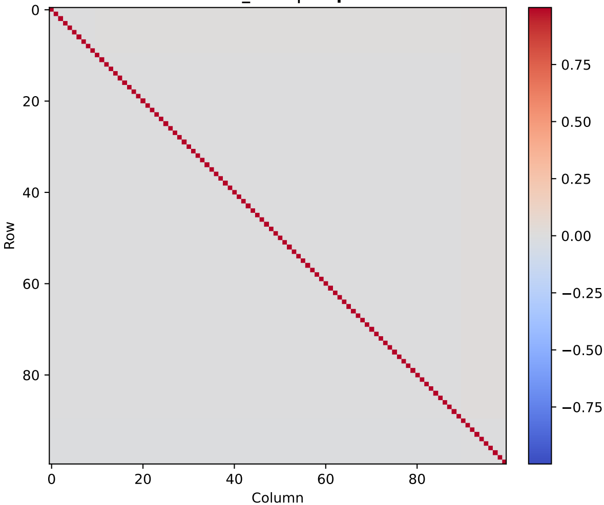
muon_zero | step 6
