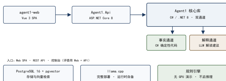
图 1 系统调用链
