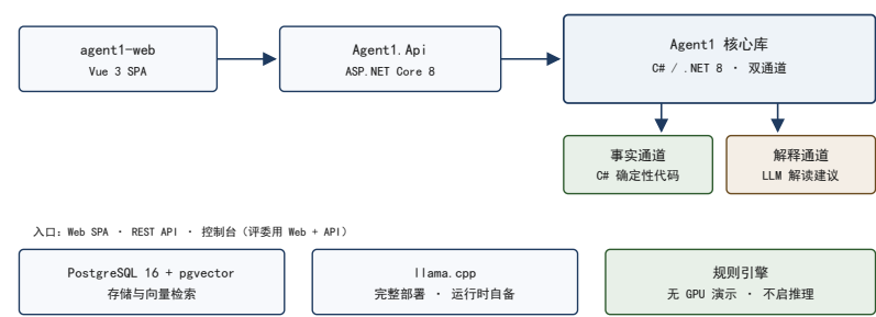
图 1 系统调用链
