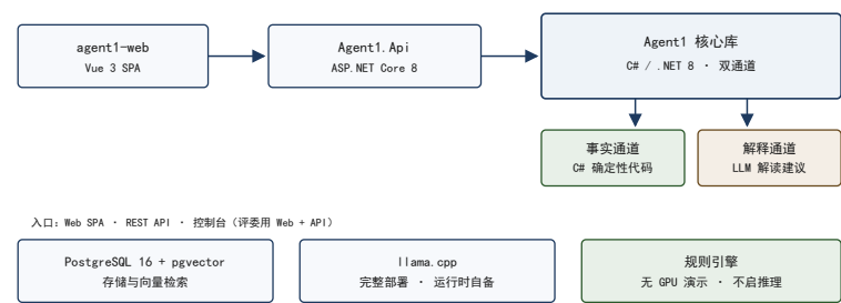
图 1 系统调用链
