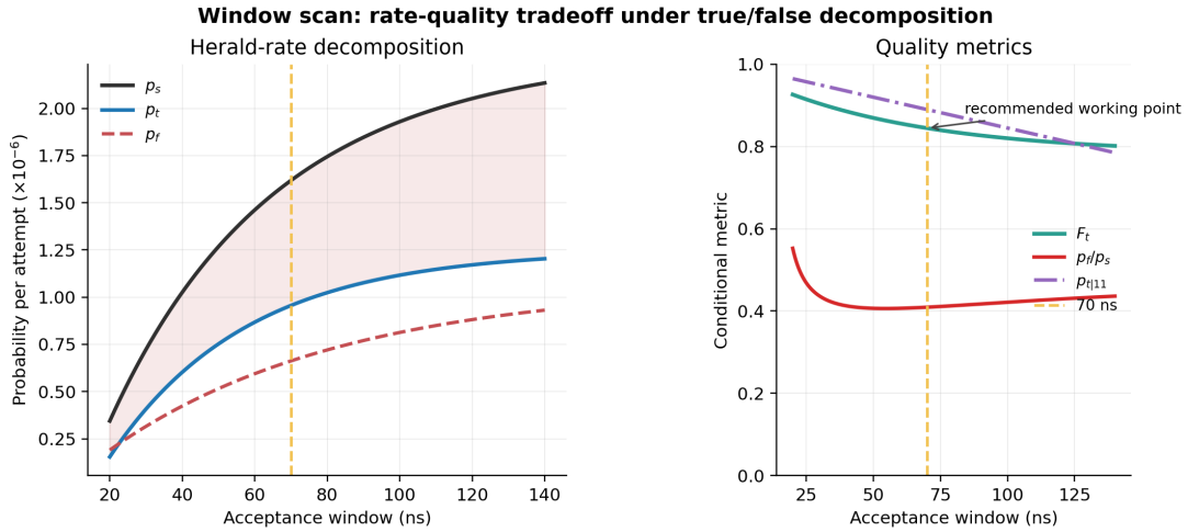
图 4-4 窗口扫描下的速率、条件保真度与假成功占比。
