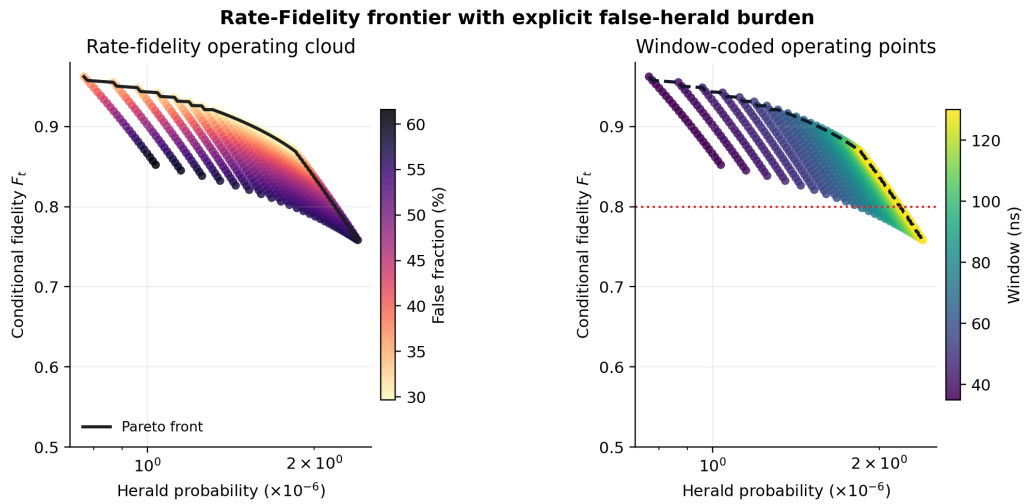
图 4-11 速率-保真度工作点前沿。
