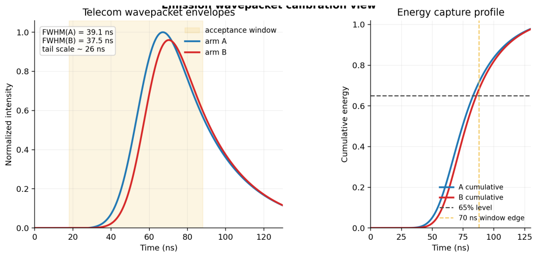
图 4-1 双臂波包时域结构与主窗口位置。
