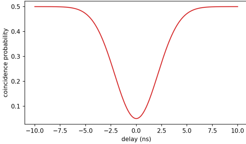
图 4-5 HOM 曲线及可见度约束。
