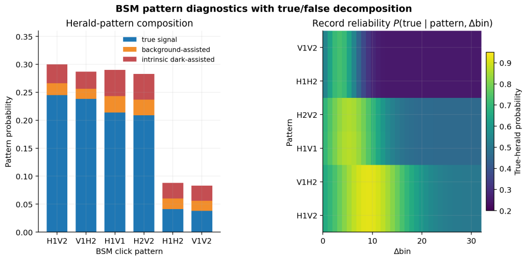
图 4-6 BSM 模式概率与真假分量分解。
