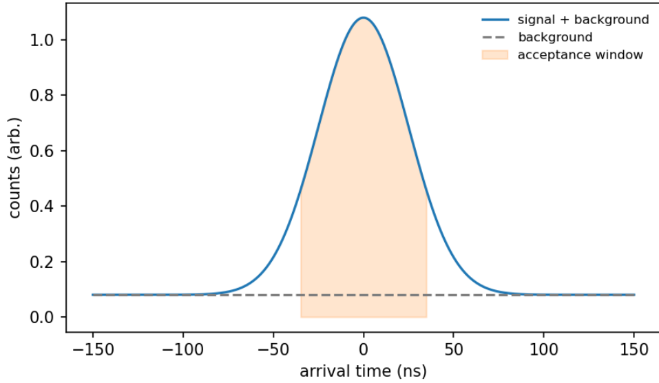
图 4-3 点击时间分布与接受窗口。
