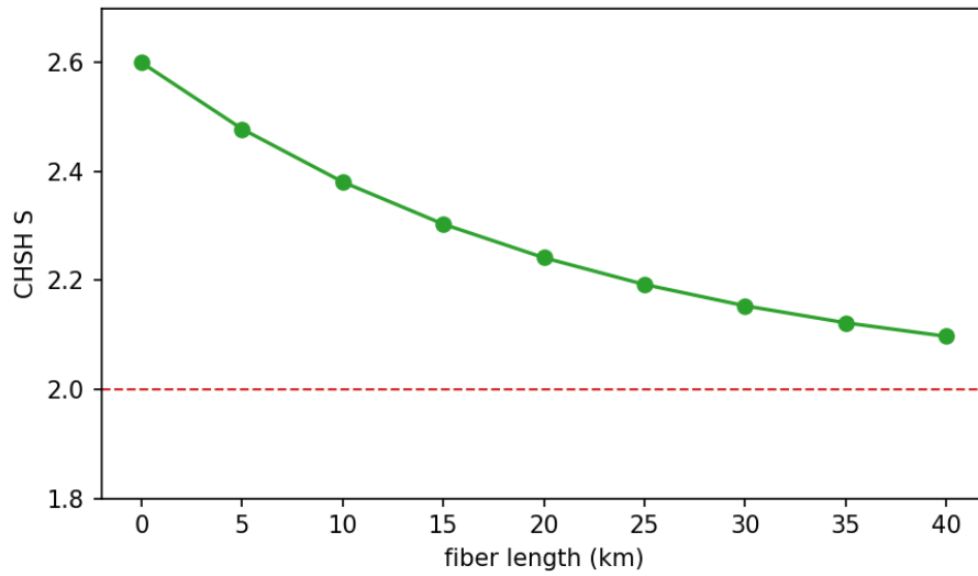
图 4-7 CHSH 参数趋势（虚线为经典界 S = 2 ）。
