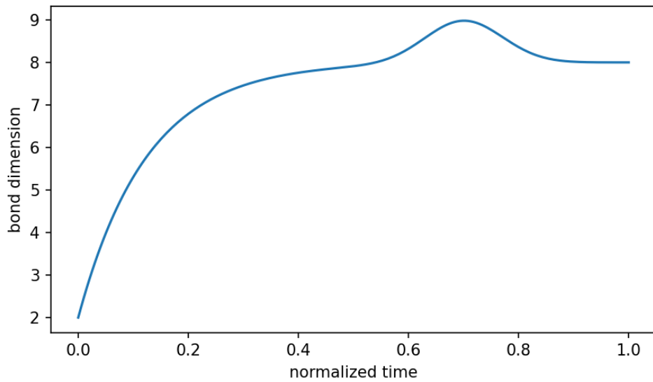
图 4-2 发射阶段 MPS 键维演化。
