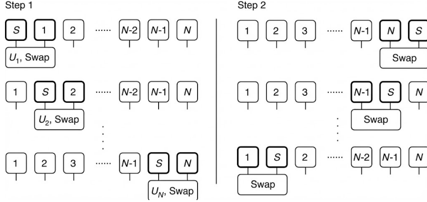
图 1-3 时间 bin 离散化与矩阵乘积态 (MPS) 更新的示意图：系统 S 与连续输出光场的相互作用被离散化为与一系列时间 bin ( B_1, B_2, \dots ) 的逐步耦合；每一步相互作用可以表示为系统与当前 bin 之间的局域幺正门，随后对已离开相互作用区的 bin 进行测量或迹掉。这种“逐 bin 更新”的结构天然适合用 MPS/TEBD 算法高效表示和演化，使得包含长时间序列光场自由度的量子态计算变得可行。 [18]
