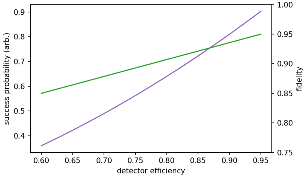
图 4-10 探测效率变化对端到端性能的影响。
