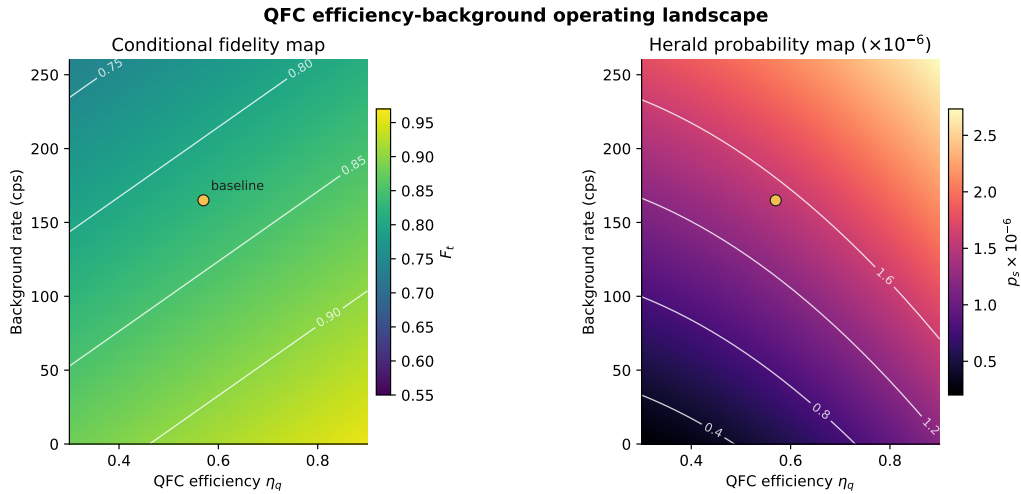
图 4-11 QFC 背景噪声对事件率与保真度的影响。
