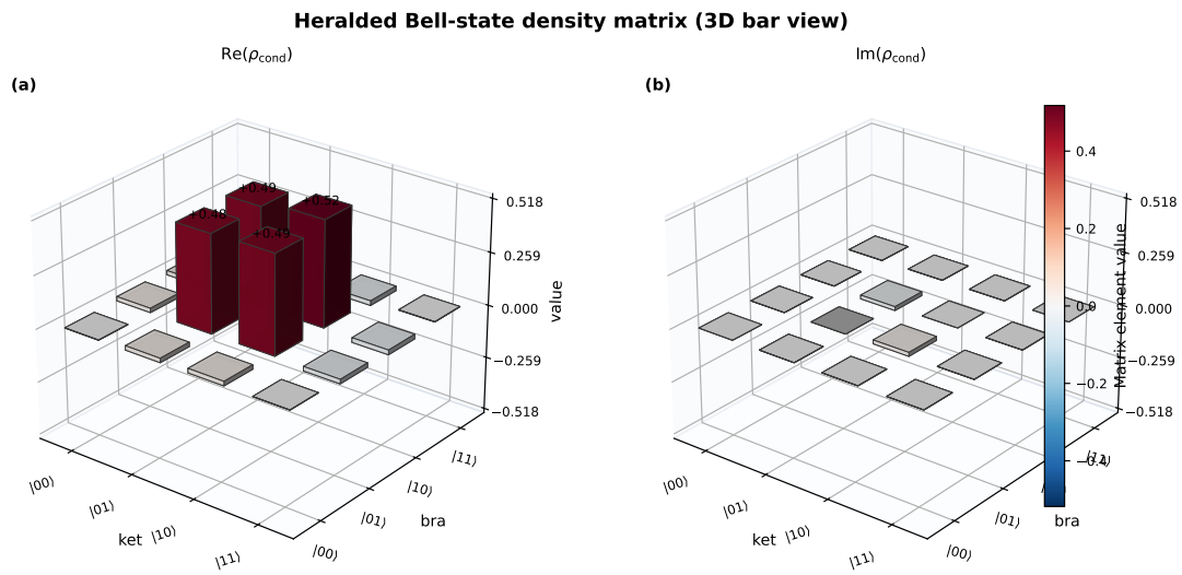
图 4-8 同一后验态的实部/虚部三维柱状图（量子信息论文常用可视化）。
