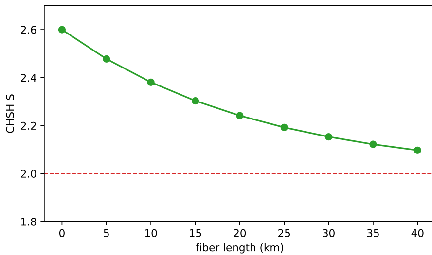
图 4-9 CHSH 参数趋势（虚线为经典界 S = 2 ）。
