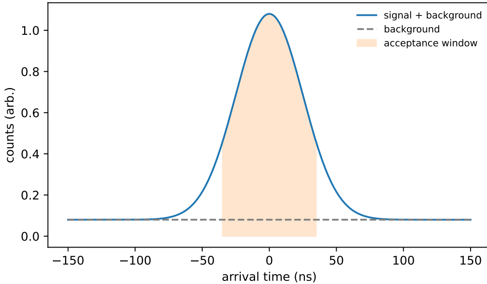
图 4-3 点击时间分布与接受窗口。
