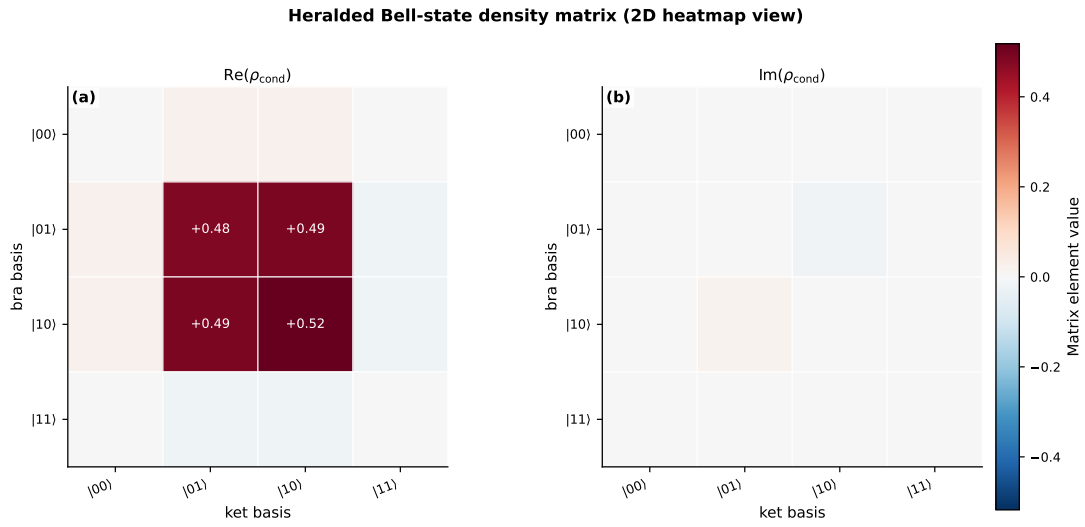
图 4-7 宣告成功条件下 Bell 后验态密度矩阵的实部/虚部二维热图。
