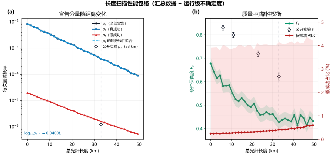
图4.8 成功率与保真度随链路长度变化。空心菱形为公开实验对照值，其中右图为6/11/23/33 km的原子-原子纠缠保真度，左图为33 km处宣告成功概率 1.22 \times 10^{-6} [29]。
