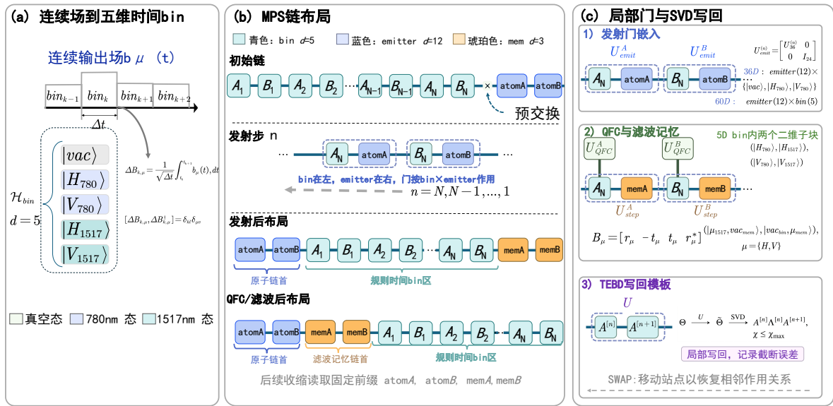
图 2.1 连续时间链路到 MPS/TEBD 计算对象的映射。连续输出场在时间步长 \Delta t 下离散为时间分箱。两臂发射体、时间分箱和滤波记忆模随后排列成一维 MPS 链。每个时间步由发射门、QFC 门、滤波记忆门、SWAP 调度和 SVD 回写组成。该结构把连续时间光场、有限带宽记忆和局域门更新统一到可收缩的张量网络表示中 [47,49,50,55-57] 。
