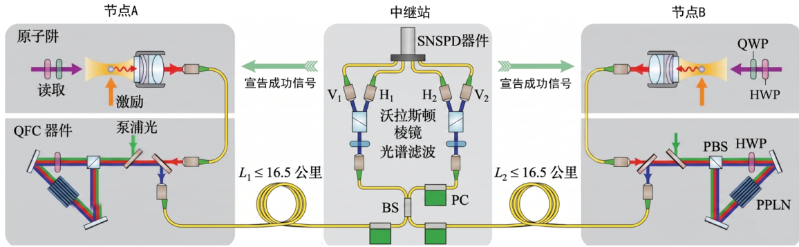
图 1.3 端到端中性原子远程纠缠链路。节点 A 和节点 B 通过读出、激发与原子-光子接口产生链路光子，QFC 模块将原子波段光子转换到电信波段并经 L_1, L_2 \leq 16.5 \text{ km} 光纤送入中继站。中继站利用沃拉斯顿棱镜、光谱滤波、分束器、偏振分析和 SNSPD 完成部分 BSM，并向两端返回成功宣告。图中“宣告成功信号”表示 heralding signal。BS 为分束器，PBS 为偏振分束器，HWP/QWP 为半波片/四分之一波片，PPLN 为周期极化铌酸锂波导，SNSPD 为超导纳米线单光子探测器 [28,29,32-34] 。
