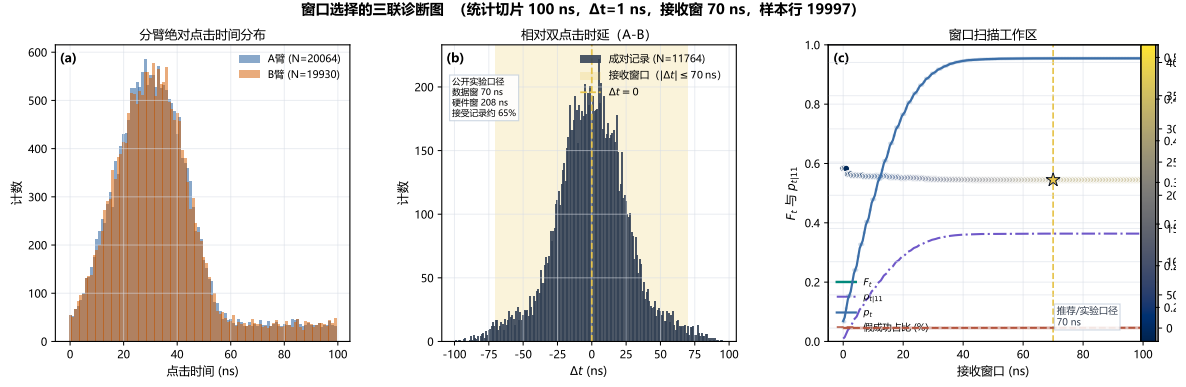
图 4.3 窗口选择的三联诊断图: (a) A/B 两臂绝对点击时间分布; (b) 相对双点击时间差分布, 其中淡黄色阴影为 \pm 70 ns 的时间差接收窗口, 并标注公开实验中的 70 ns 数据窗口、208 ns 硬件符合窗口和约 65% 接受比例; (c) 窗口扫描下的工作区, 同时给出 F_t 、 p_{t|11} 、 p_t 与假成功占比 [29] 。
