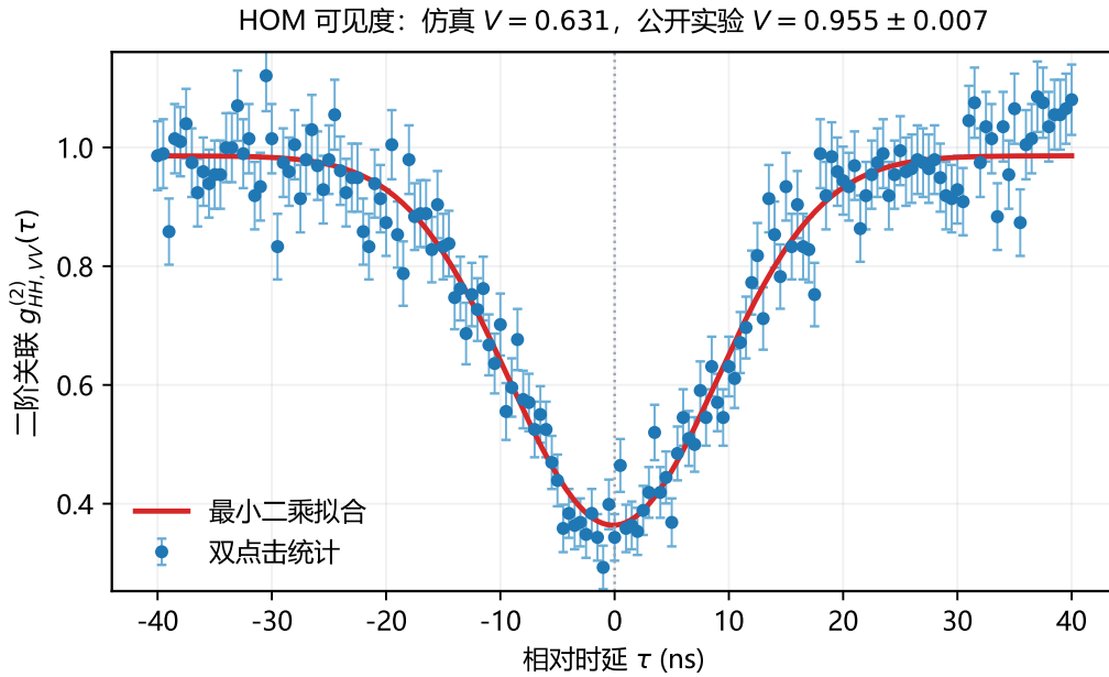
图 4.4 基于同偏振跨端口双点击统计的 HOM 二阶关联曲线及最小二乘拟合。标题同时给出端到端仿真拟合得到的 HOM 可见度和公开实验可见度 0.955(7) [29] 。
