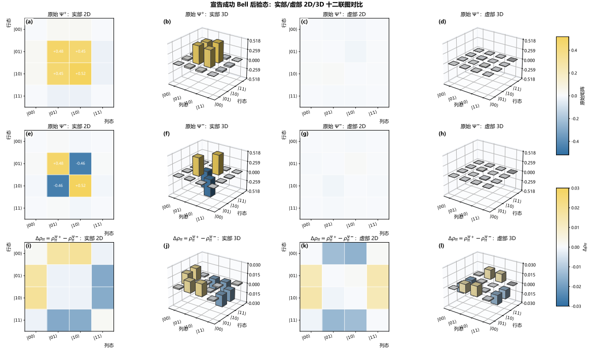
图 4.6 宣告成功条件下贝尔后验态密度矩阵的十二联图：三行分别对应原始 \Psi^+ 、原始 \Psi^- 与 \Delta\rho_{\text{Bell}} = \rho_{\text{Bell}}^{\Psi^+} - \rho_{\text{Bell}}^{\Psi^-} 。每行四列依次为二维实部热图、三维实部柱图、二维虚部热图与三维虚部柱图。
