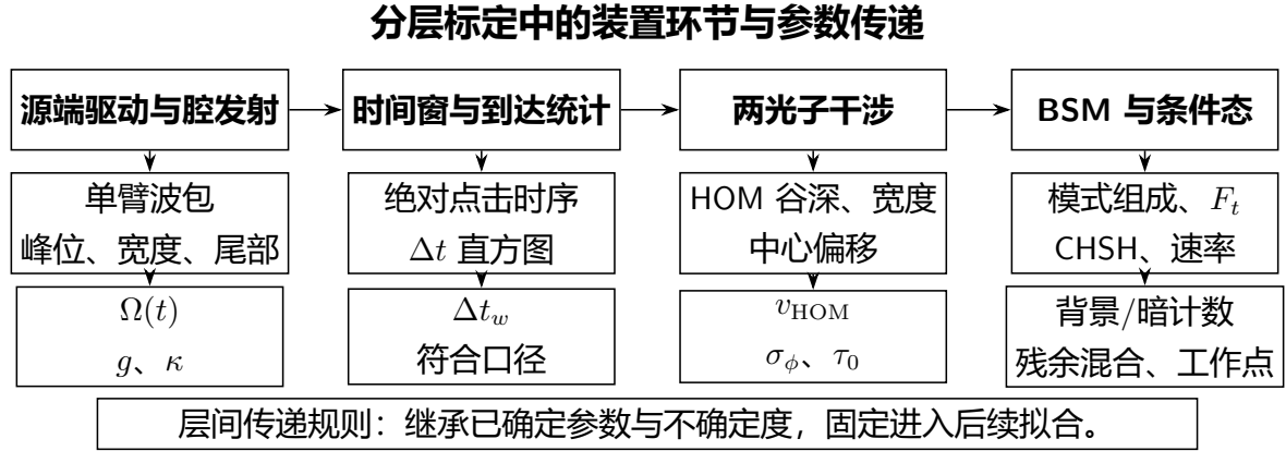
图 4.1 按装置环节组织的分层标定图：从源端发射、时间窗、HOM 干涉到 BSM 与条件态，每一层只用本层观测锚定对应参数，并把约束传递到下一层。
