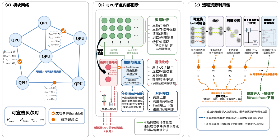
图 1.2 模块化量子处理网络的资源架构。多个 QPU 节点通过可宣告远程 Bell 对形成网络边。节点内部由承担本地门、存储、读出和综合征循环的数据比特，以及承担原子-光子接口的通信比特共同组成。远程 Bell 对带有保真度、建立速率、宣告延迟和成功记录等资源指标，并可经纯化、纠缠交换和门传送进入跨模块门或逻辑操作。
