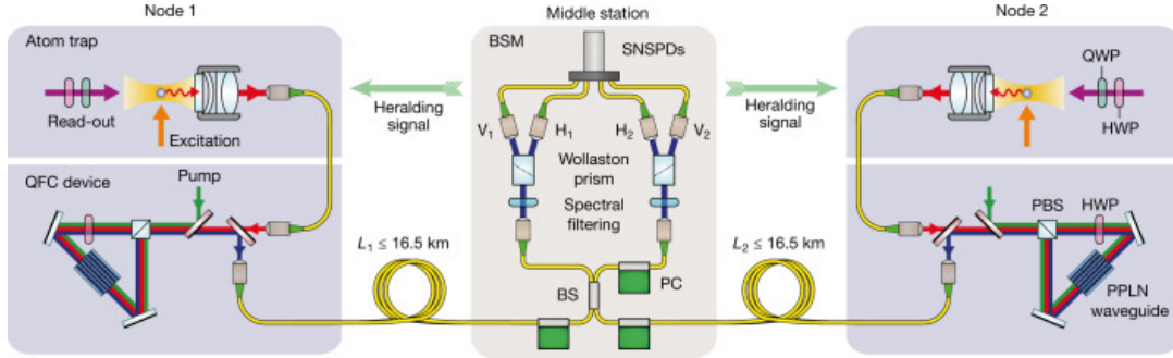
图 1-2 面向中性原子处理节点的光子-原子量子接口典型链路示意：两端各有一个被光镊囚禁的单个 ^{87}\text{Rb} 原子，通过受激拉曼绝热转移（stimulated Raman adiabatic passage, STIRAP）产生原子-光子纠缠；780 nm 光子经 QFC 转换到电信波段（1517 nm）后进入长光纤链路，在中继站进行两光子干涉与 BSM；符合点击作为“宣告信号”将远程原子寄存器投影到纠缠态。
