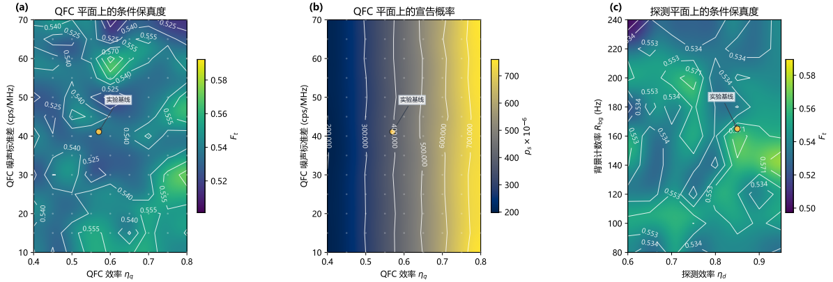
图 4.9 器件参数工作平面：(a) QFC 效率与背景噪声对应的条件保真度热图；(b) 同一 QFC 参数平面上的宣告概率热图；(c) 探测效率与背景计数对应的条件保真度热图。金色圆点表示由公开实验器件参数给出的基线锚点，包含 \eta_q = 0.57 、 \eta_d \gtrsim 0.85 和 R_{bg} \sim 160\text{--}170\text{ s}^{-1} 的量级 [28-29]。
