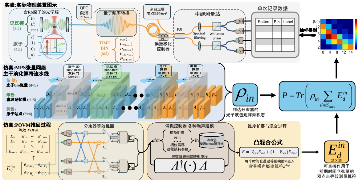
图 3.2 端到端单次任务仿真流程图。状态侧负责发射 TEBD、QFC、滤波记忆和原子退相干，并生成切分面输入态 \rho_{\text{in}} 。测量侧负责光纤、分束器、探测器 POVM、背景事件、成功模式枚举和输入端效应 E_m^{\text{in}} 构造。两条数据流在条件化收缩中合并，输出宣告概率、条件态和第四章指标入口 [47,49]。
