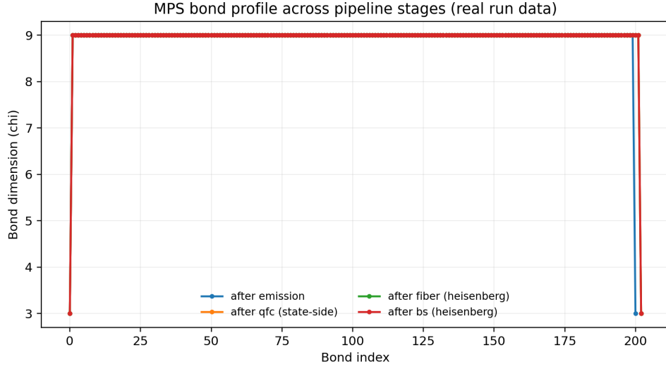
图 4-3 发射阶段 MPS 键维演化。
