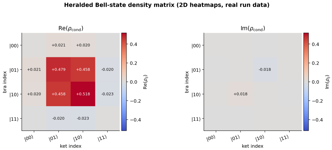
图 4-8 宣告成功条件下 Bell 后验态密度矩阵的实部/虚部二维热图。
