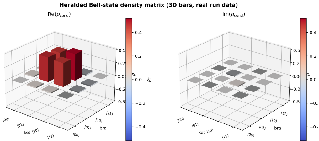
图 4-9 同一后验态的实部/虚部三维柱状图（量子信息论文常用可视化）。
