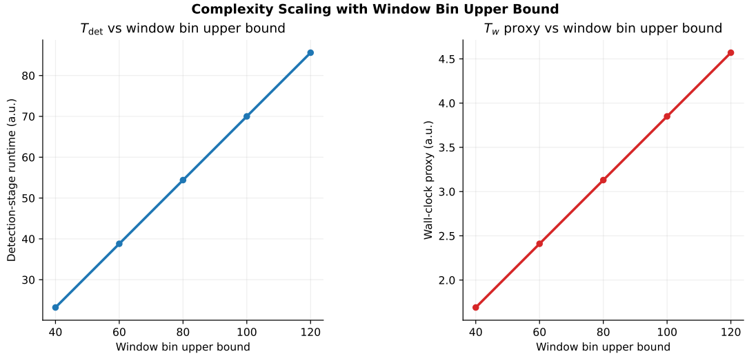
图 4-15 复杂度缩放图：左为探测阶段耗时随窗口 bin 数增长，右为墙钟代理量随 bin 个数上限增长。
