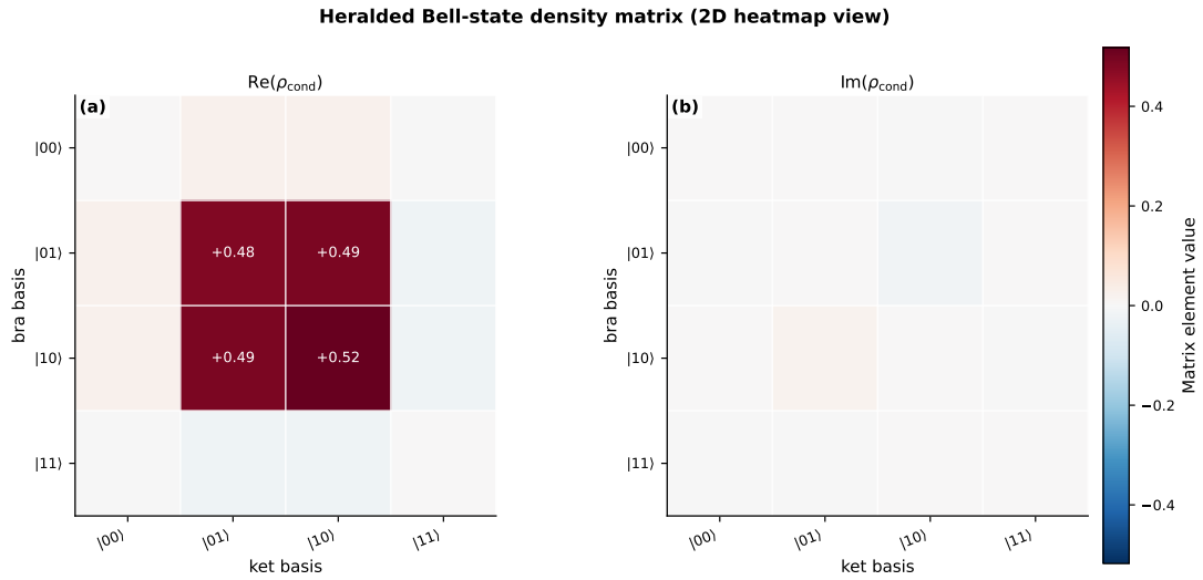
图 4-7 宣告成功条件下 Bell 后验态密度矩阵的实部/虚部二维热图。
