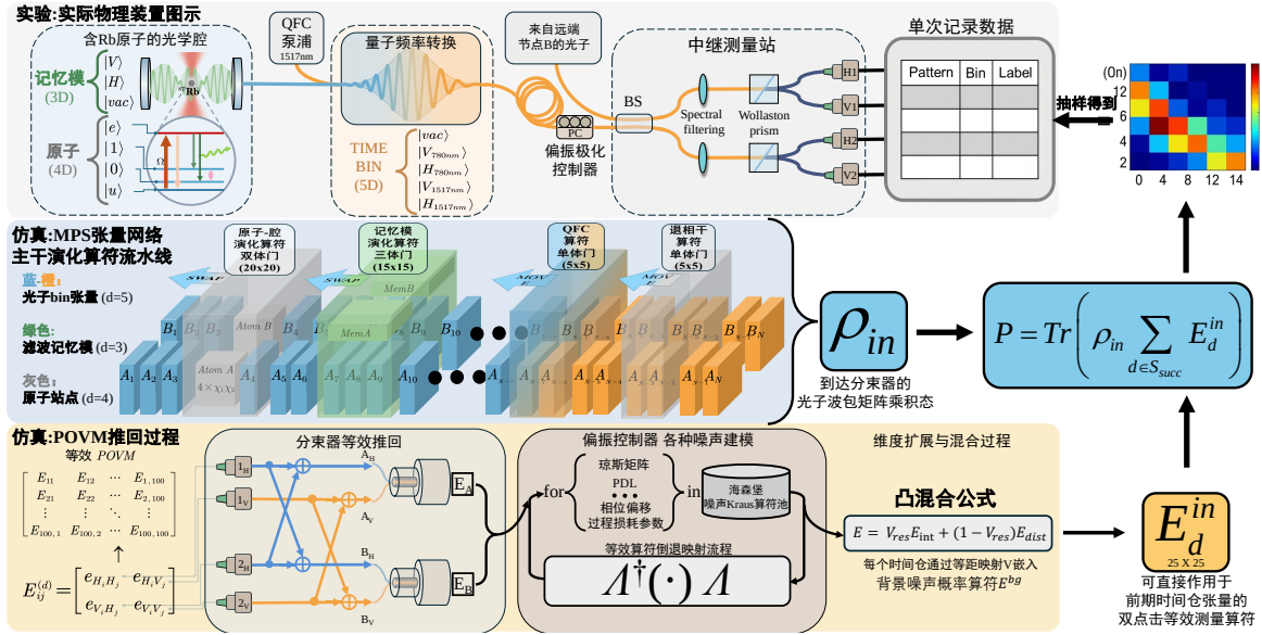
图 3.2 单链路仿真任务流程图。状态侧负责发射 TEBD、QFC、滤波记忆和原子退相干，并生成切分面输入态 \rho_{\text{in}} 。测量侧负责光纤、分束器、探测器 POVM、背景事件、成功模式枚举和输入端效应 E_m^{\text{in}} 构造。两条数据流在条件化收缩中合并，输出宣告概率、条件态和第四章指标入口。
