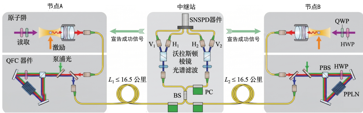
图 1.3 中性原子远程纠缠链路。节点 A 和节点 B 通过读出、激发与原子-光子接口产生链路光子, QFC 模块将原子波段光子转换到电信波段并经 L_1, L_2 \leq 16.5 \text{ km} 光纤送入中继站。中继站利用沃拉斯顿棱镜、光谱滤波、分束器、偏振分析和 SNSPD 完成部分 BSM, 并向两端返回成功宣告。图中“宣告成功信号”表示中继站返回两端节点的经典宣告信号。BS 为分束器, PBS 为偏振分束器, HWP/QWP 为半波片/四分之一波片, PPLN 为周期极化铌酸锂波导, SNSPD 为超导纳米线单光子探测器 [29,30,36,38,39] 。
