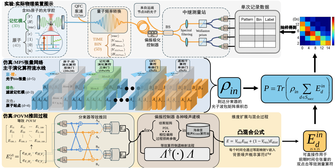
图 3.2 单次链路仿真任务流程图。状态侧负责发射 TEBD、QFC、滤波记忆和原子退相干，并生成切分面输入态 \rho_{in} 。测量侧负责光纤、分束器、探测器 POVM、背景事件、成功模式枚举和输入端效应 E_m^{in} 构造。两条数据流在条件化收缩中合并，输出宣告概率、条件态和第四章指标入口。
