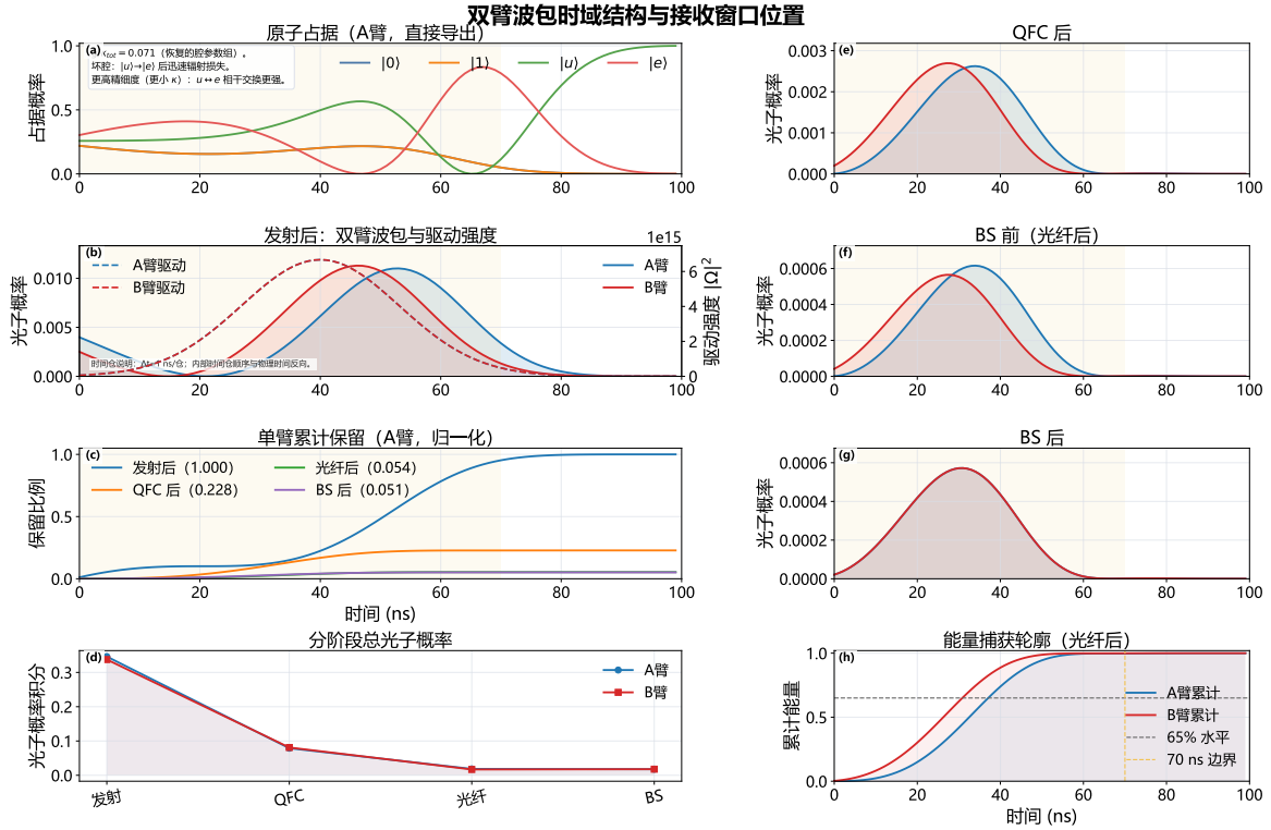
图 4.2 双臂波包时域结构与主窗口位置：(a) A 臂原子四能级占据演化；(b) 发射后双臂波包；(c) A 臂累计保留率；(d) 各阶段总光子概率积分；(e) QFC 后双臂波包；(f) 光纤后、入分束器前波包；(g) 分束器后波包；(h) 光纤后累计能量捕获。
