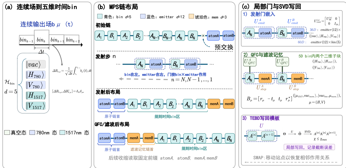
图 2.1 连续时间链路到 MPS/TEBD 计算对象的映射。连续输出场在时间步长 \Delta t 下离散为时间分箱。两臂发射体、时间分箱和滤波记忆模随后排列成一维 MPS 链。每个时间步由发射门、QFC 门、滤波记忆门、SWAP 调度和 SVD 回写组成。该结构把连续时间光场、有限带宽记忆和局域门更新统一到可收缩的张量网络表示中 [47,49,50,53-55] 。
