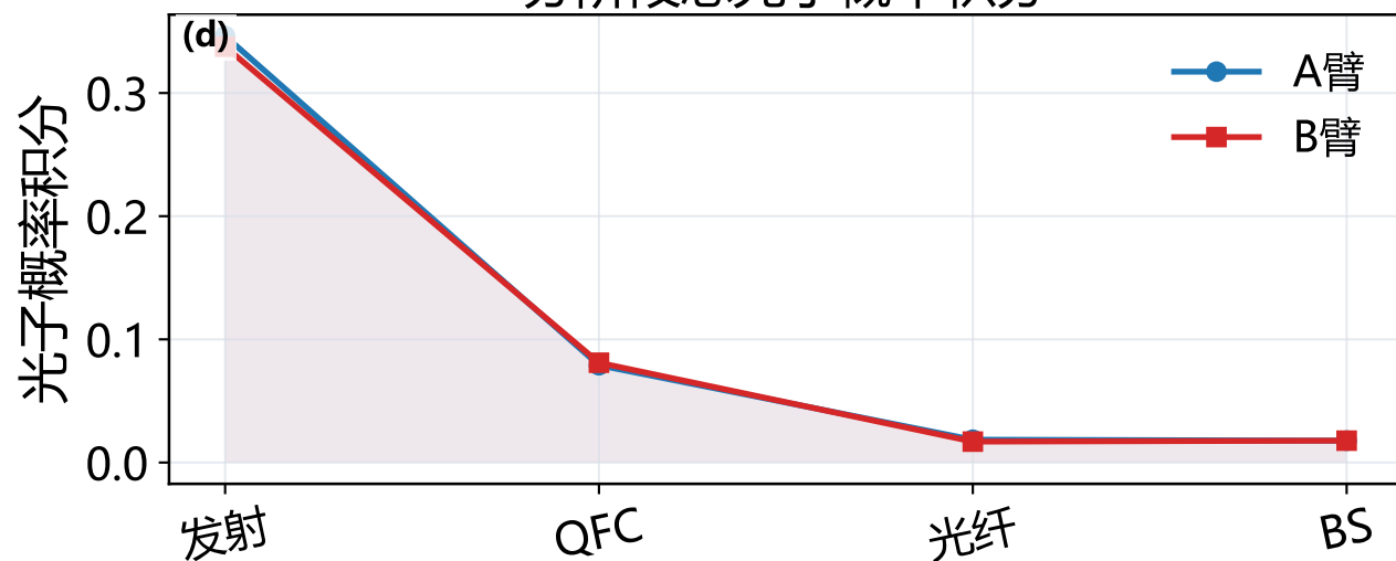
分阶段总光子概率积分
