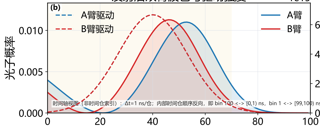
发射后双臂波包与驱动强度
