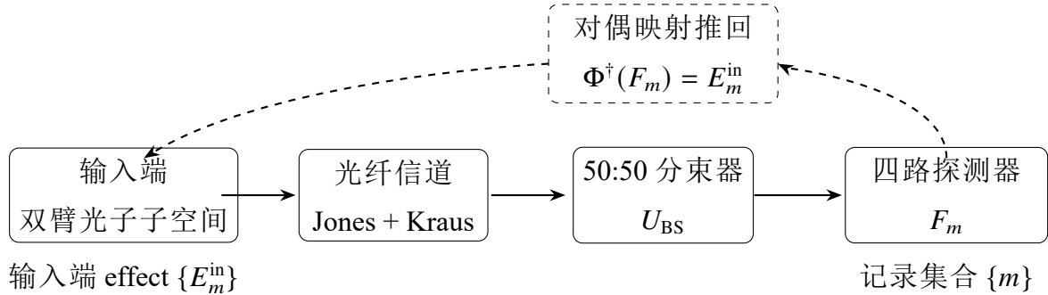
图 3.2 中间站测量侧的 effect 推回关系。探测端先构造点击记录 F_m ，再经光纤信道和分束器的对偶映射推回输入端，得到用于收缩的 E_m^{\text{in}} 。这一路径保留了损耗、偏振旋转和探测器响应，又避免在态端重复施加线性光学网络。该处理与开放系统中的对偶信道表述一致 [53,65-66] 。
